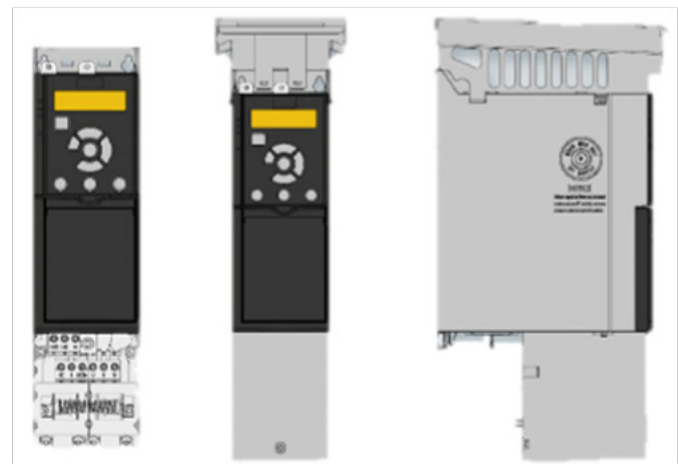
Ilustración 26: Componentes del convertidor con kit de conversión
