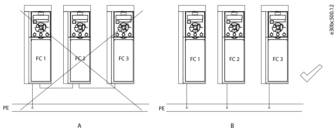
Ilustración 29: Igualización de potencial de conexión a tierra
