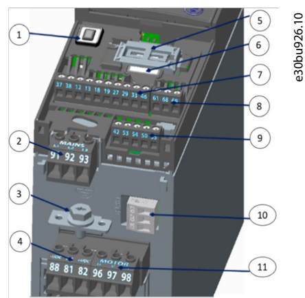
Ilustración 35: Números de los terminales
