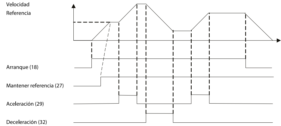
Ilustración 36: Aceleración/deceleración
