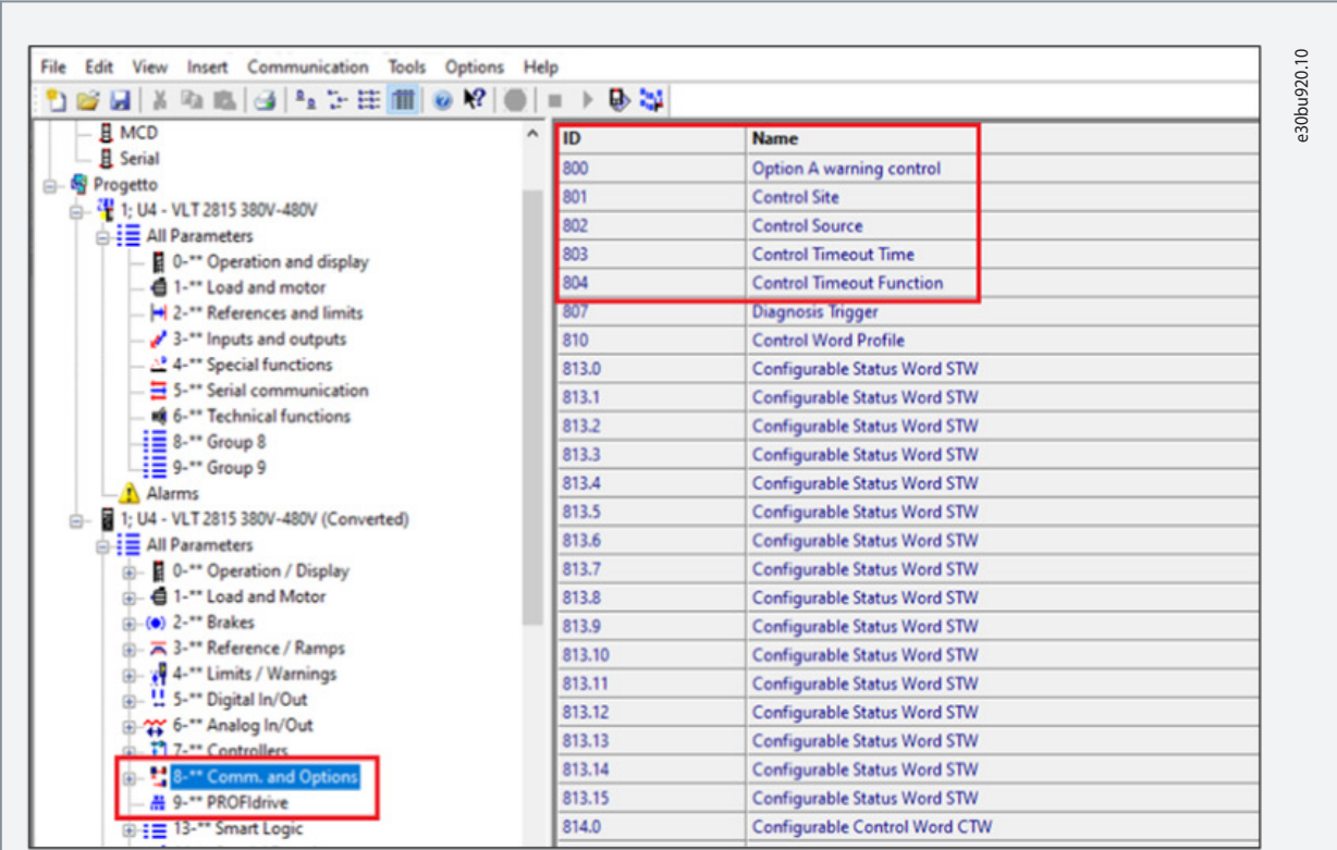
Ilustración 49: Comunic. y opciones
