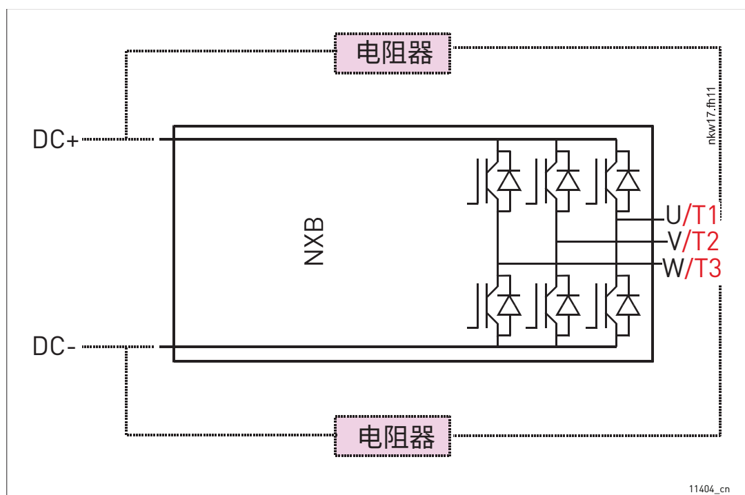
图 125. VACON® 制动斩波器单元连接
