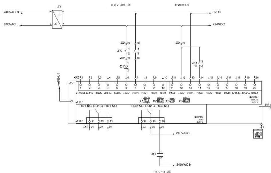
图 112. 控制单元接线图
