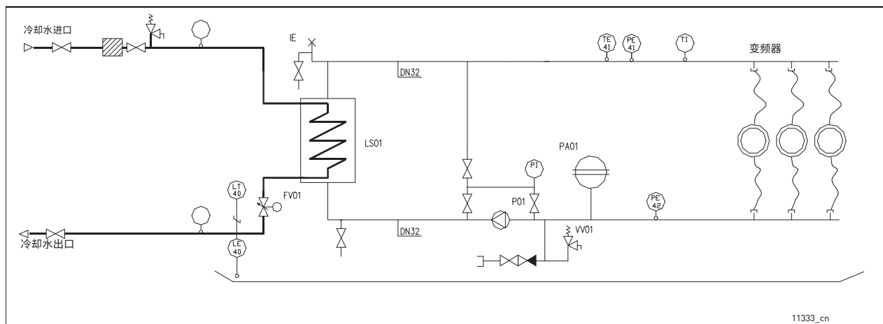
图 34. 示例：冷却系统的PI图和连接
