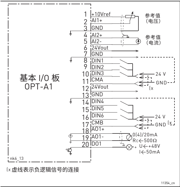
图 61. 基本 I/O 板 (OPT-A1) 的一般接线图
