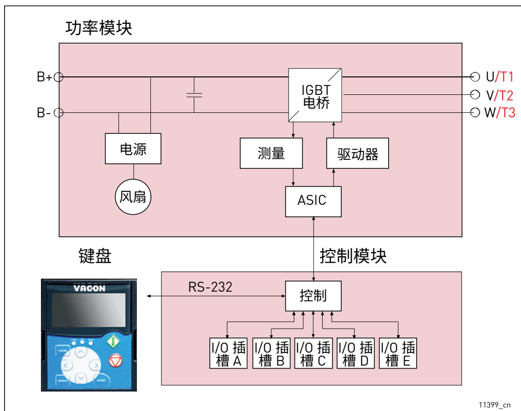
图 103. 有源前端模块示意图
