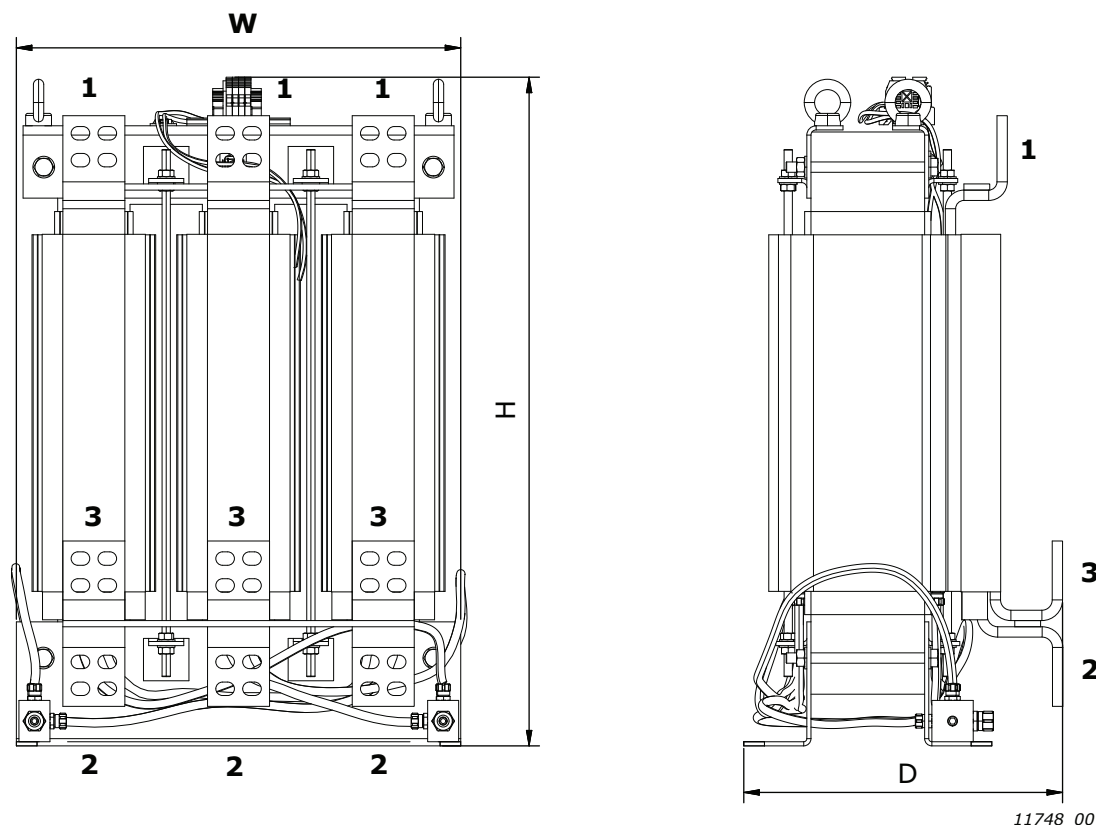
图 122. FLU-CHK-1030-6-DL 电抗器示例
