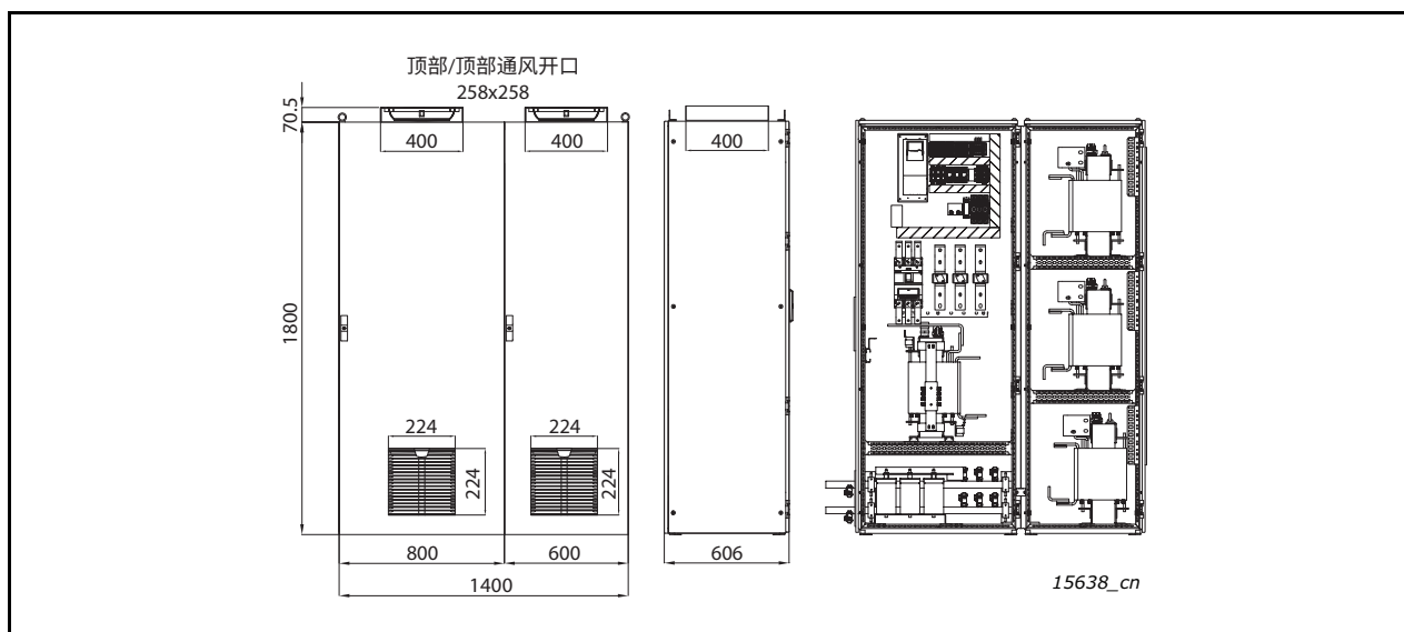
图 128. 安装在机箱中的 RLC 920 A 的布局
