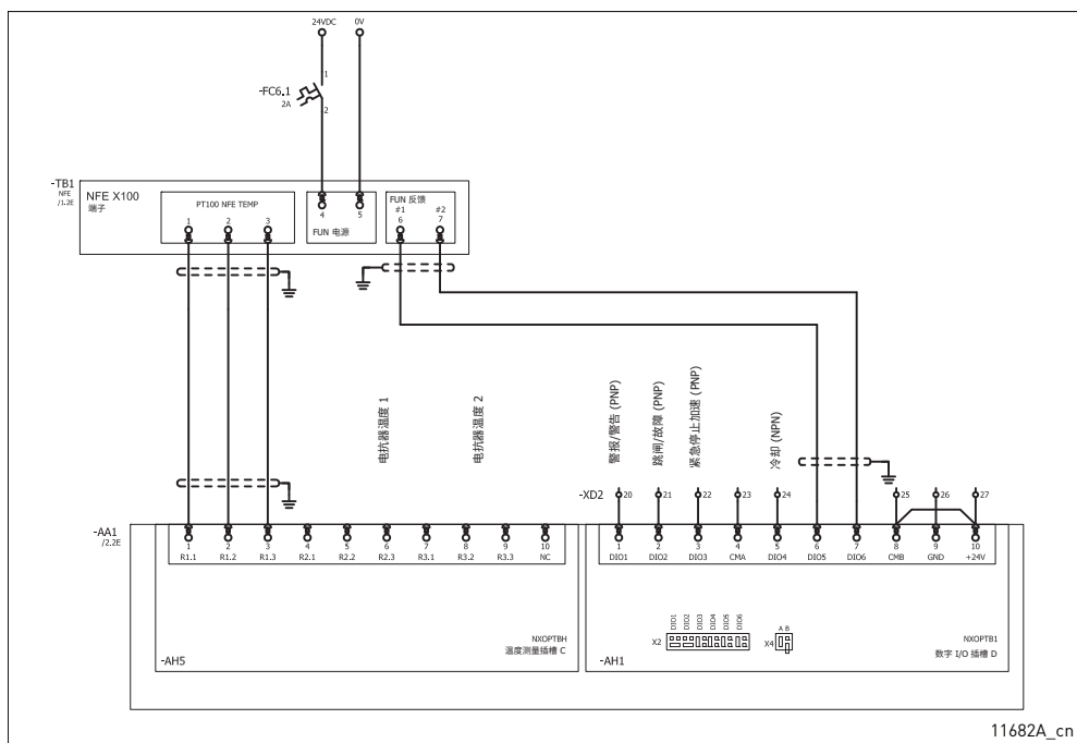
图 117. 控制装置接线图, OPTBH、OPTB1
