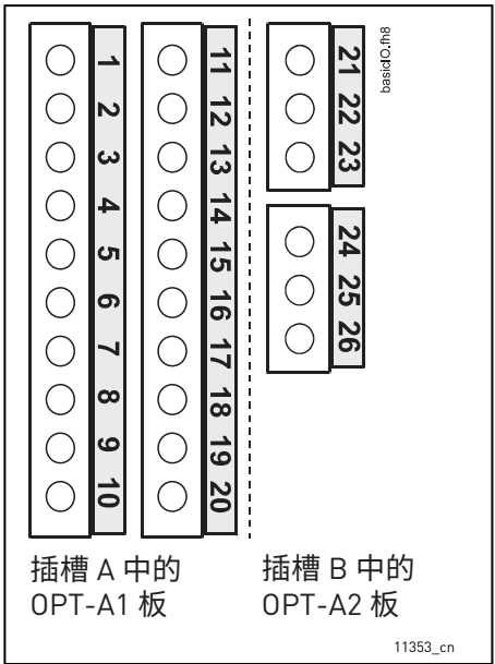
图 60. 两个基本板的 I/O 端子
