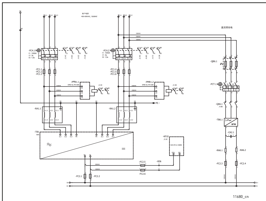
图 115. NFE 单元接线图
