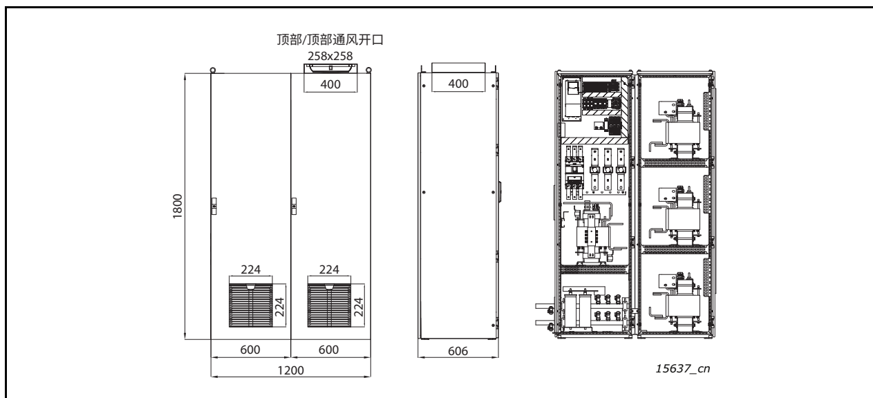
图 127. 安装在机箱中的 RLC 385/520/750 A 的布局
