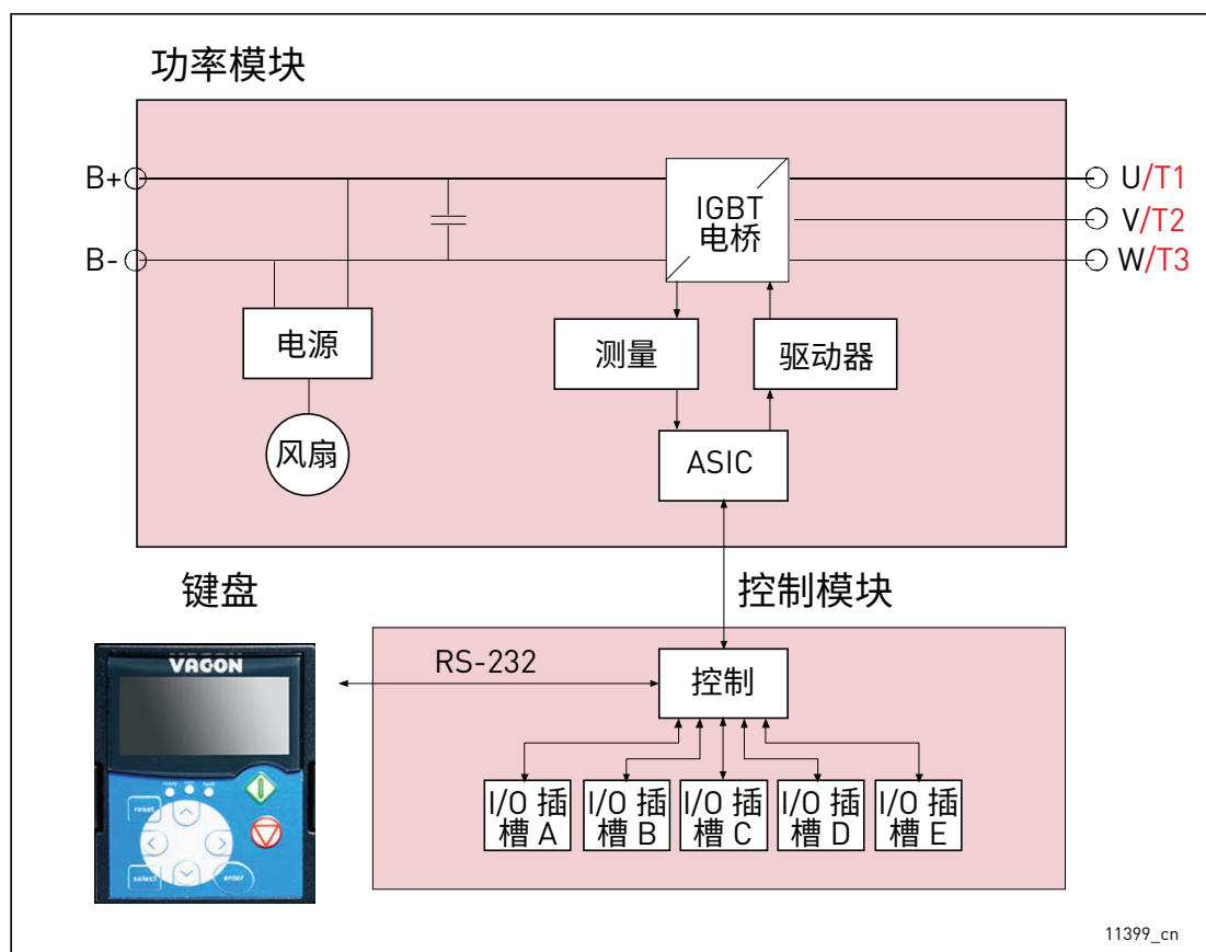
图 123. BCU 块示意图
