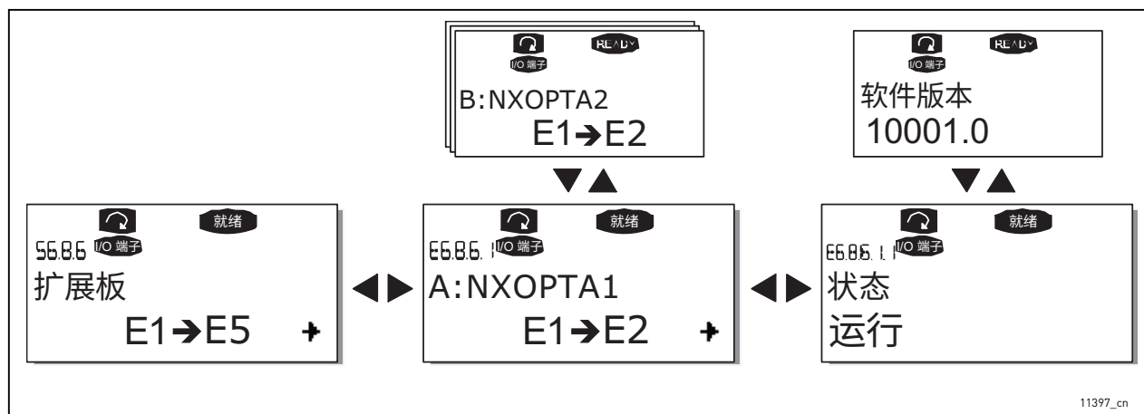
图 100. 扩展板信息菜单
