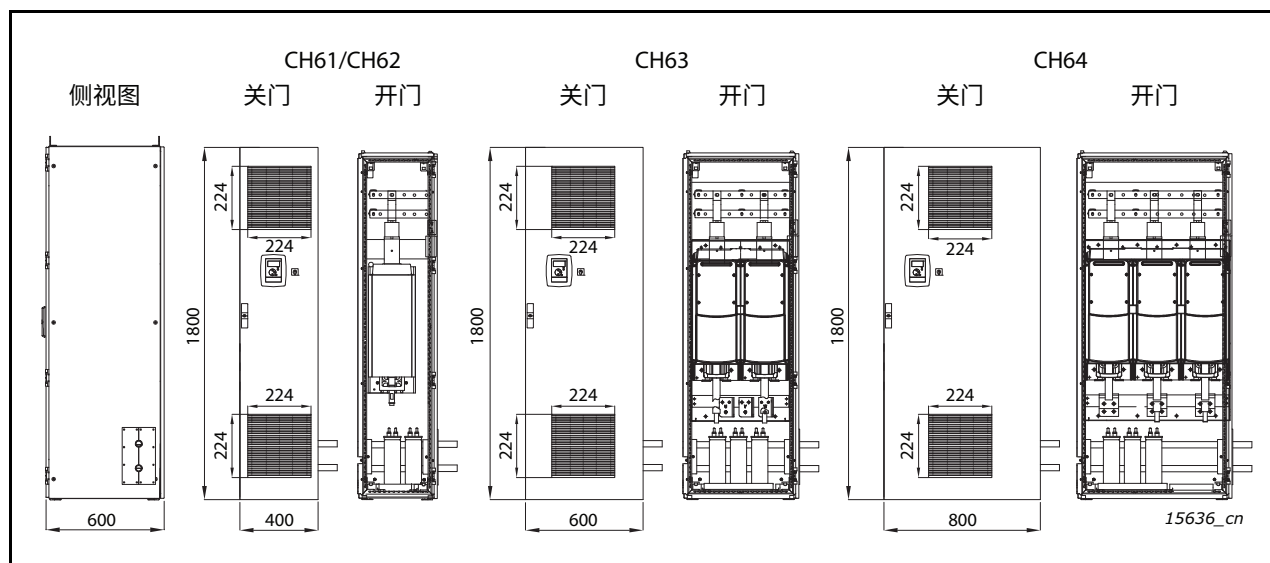
图 126. 安装在机箱中的水冷逆变器的布局
