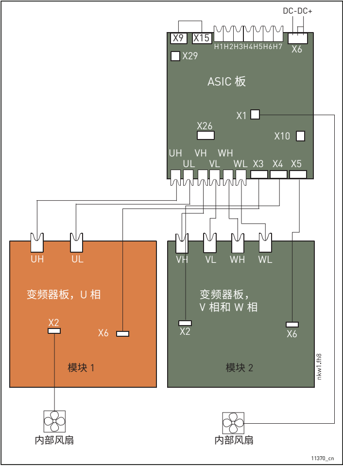
图 70. ASIC 和变频器板 (CH63) 之间的端子和连接
