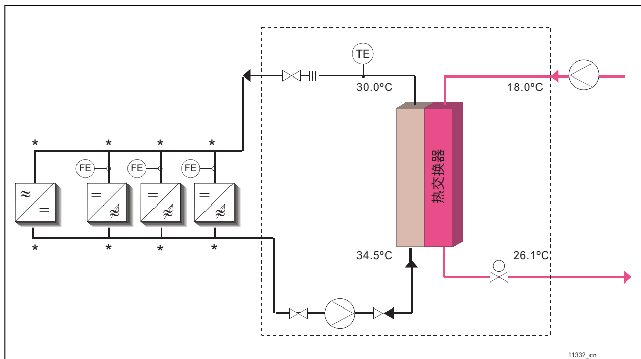
图 33. 冷却系统示例
