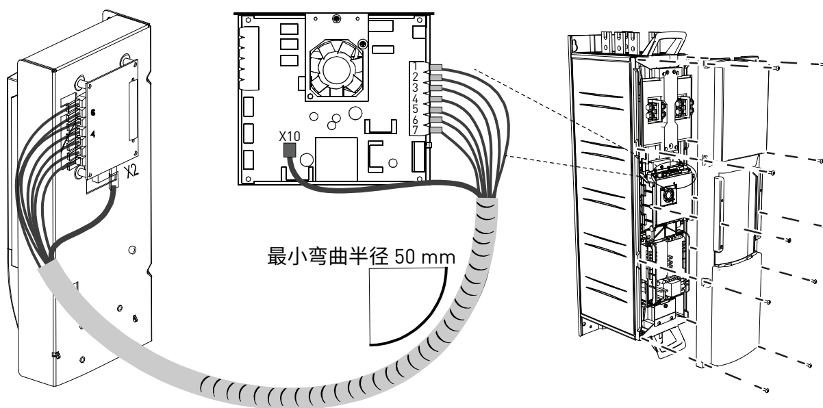
图 74. 将电源和控制电缆连接到控制单元，Ch7x
