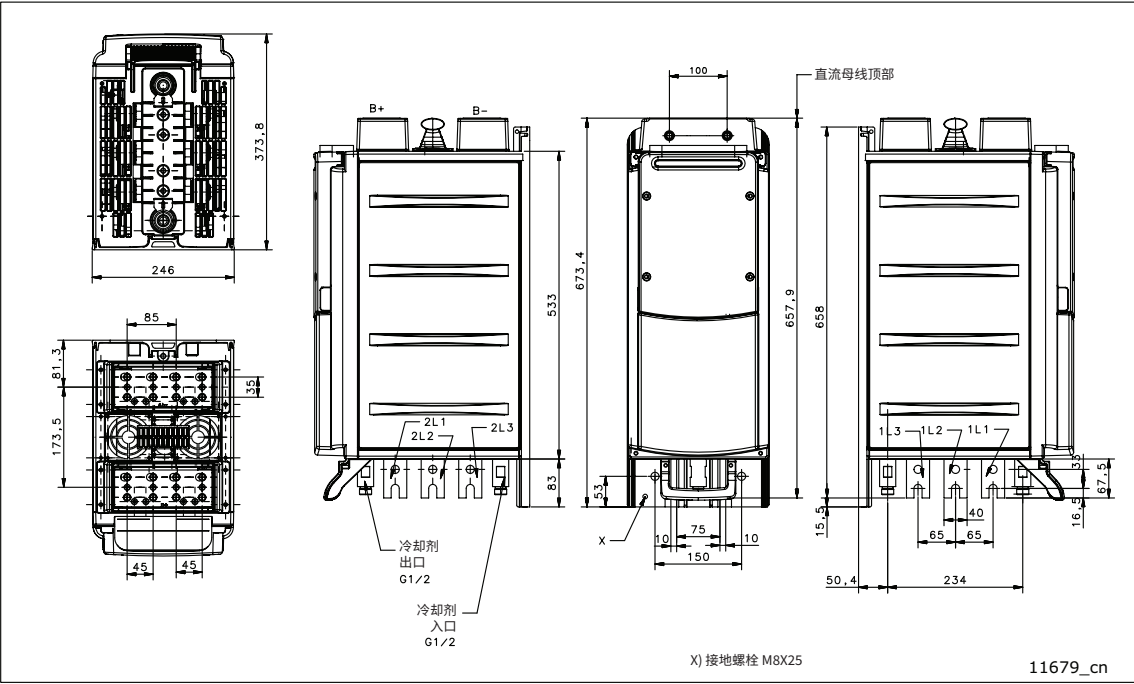
图 120. VACON® 水冷式非再生前端，CH60
