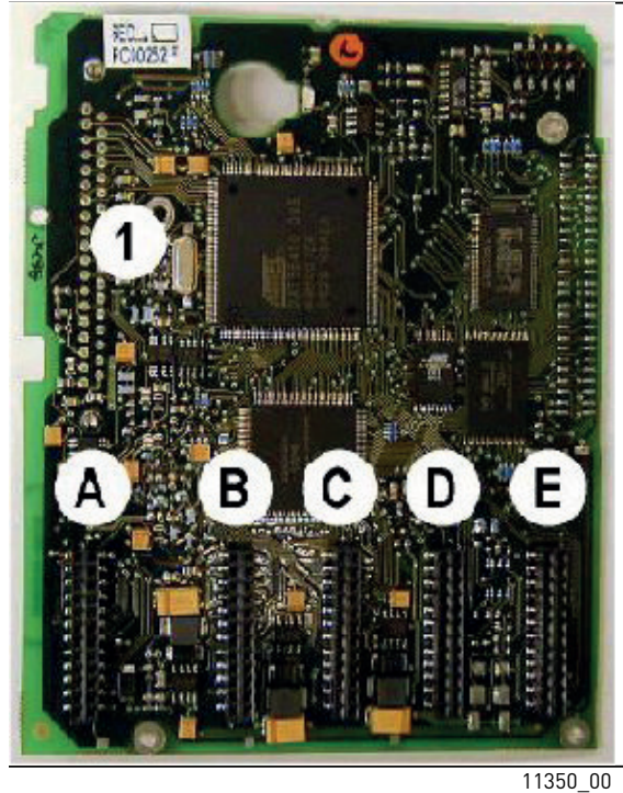
图 58. VACON® NX 控制板
