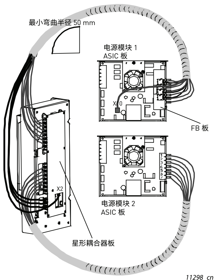
图 75. 将电源和控制电缆连接到控制单元，2xCh64 和 2xCH74
