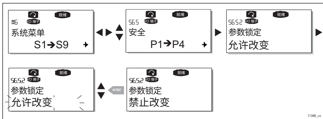
图 91. 参数锁定
