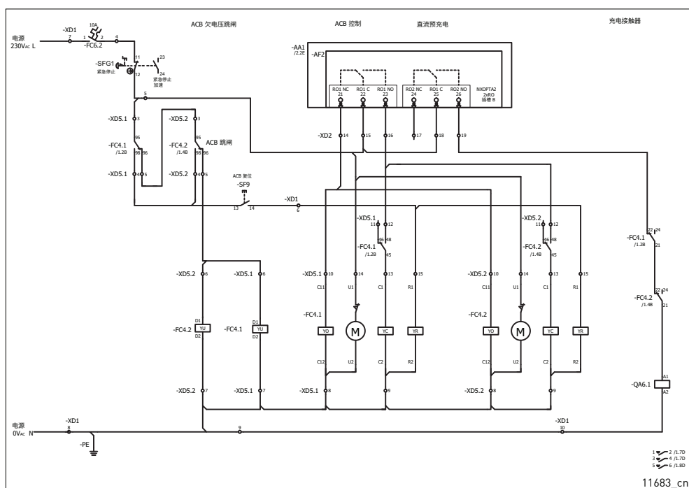
图 118. 控制装置接线图, OPTA2。
