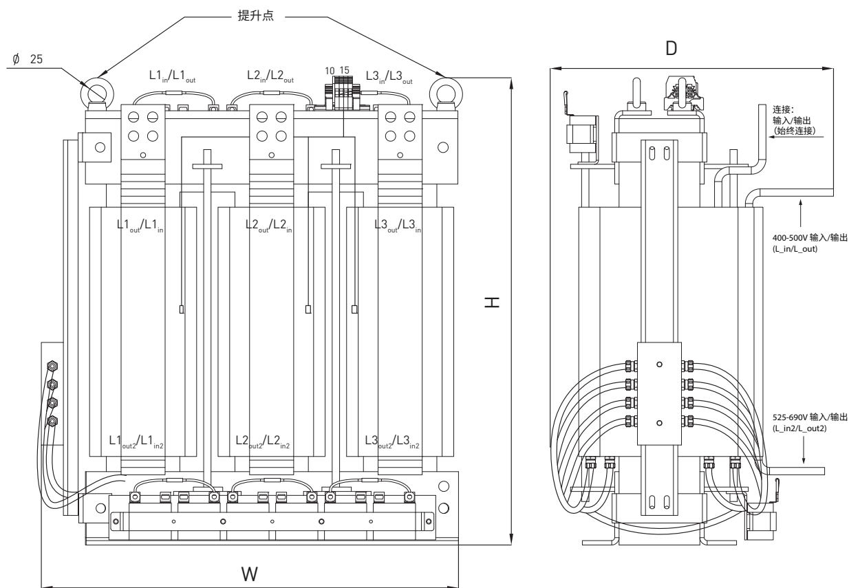
图 105. VACON® RLC 滤波器的 L_{net} 电抗器示例
