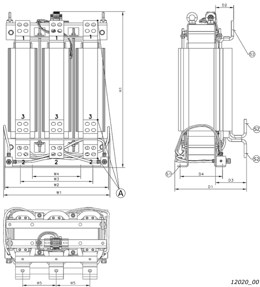
图 38. VACON® NX 水冷式变频器的水冷式输入电抗器示例。规格 261 A...1150 A
