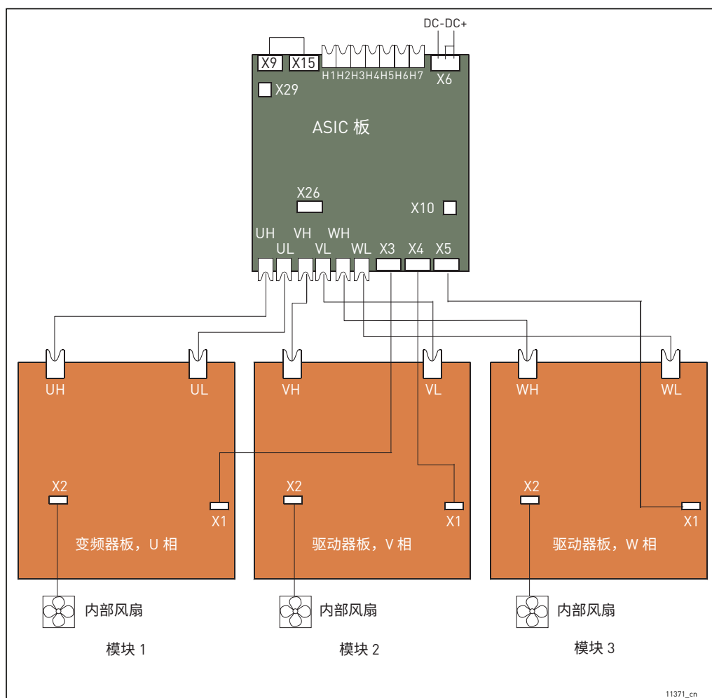
图 71. ASIC 和变频器板 (CH64 和 CH74) 之间的端子和连接
