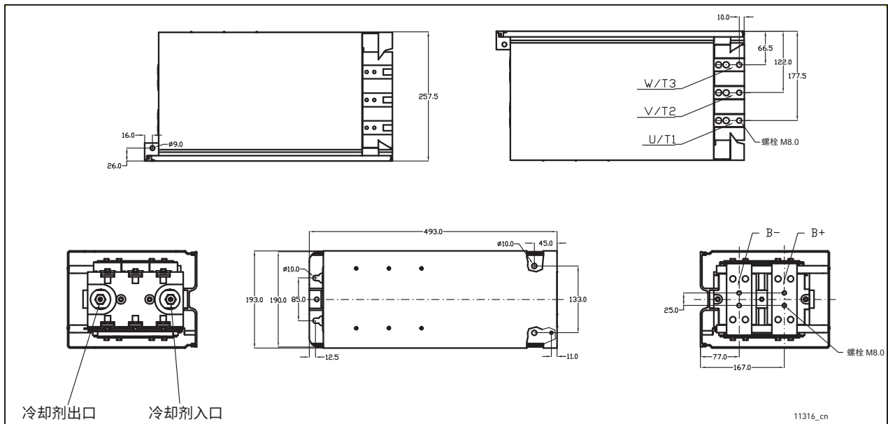
图 9. VACON® NX 水冷式变频器尺寸 (逆变器), CH4
