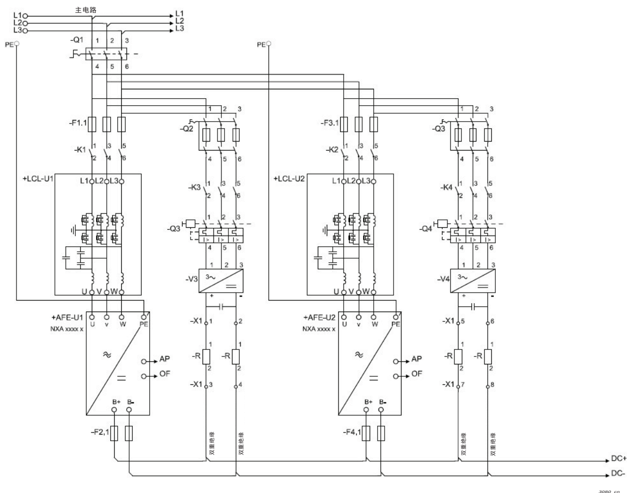
图 114. 有源前端单元与各自的预充电电路并联
