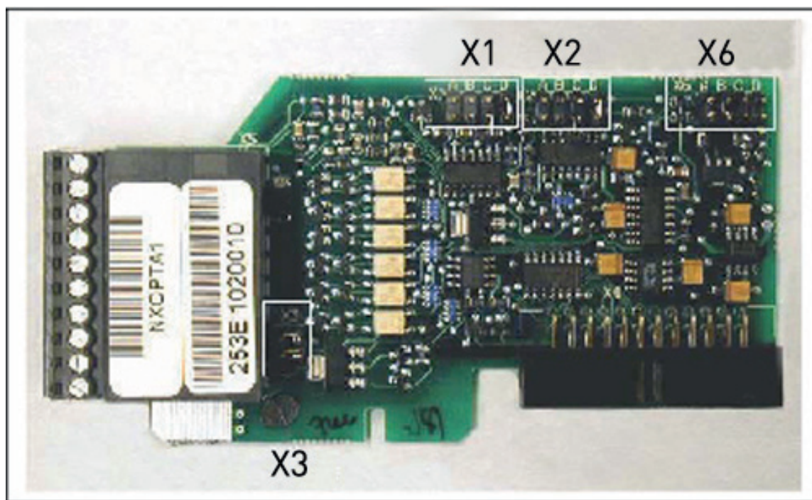
图 65. OPT-A1 上的跳线块
