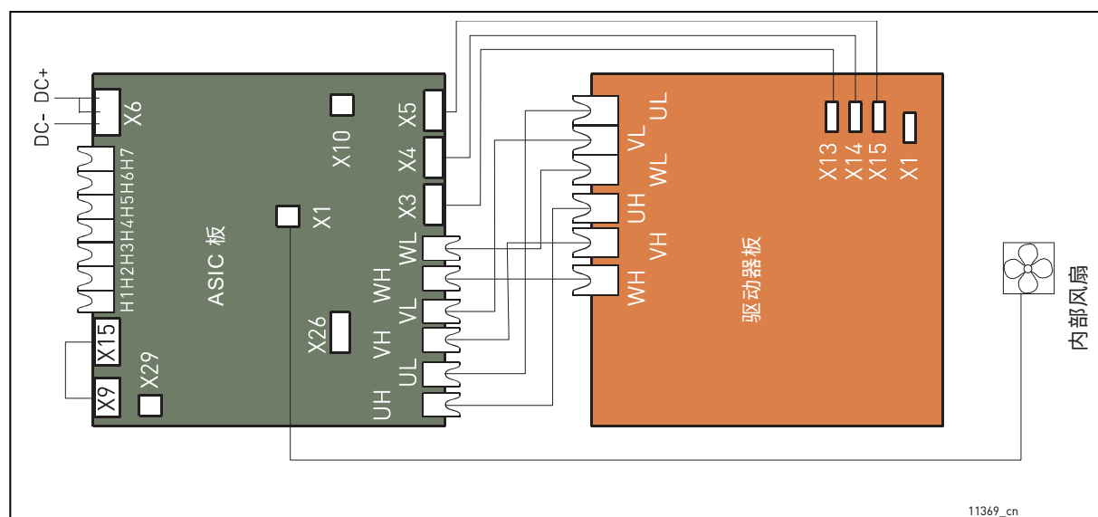
图 69. ASIC 和变频器板 (CH61、CH62 和 CH72) 之间的端子和连接
