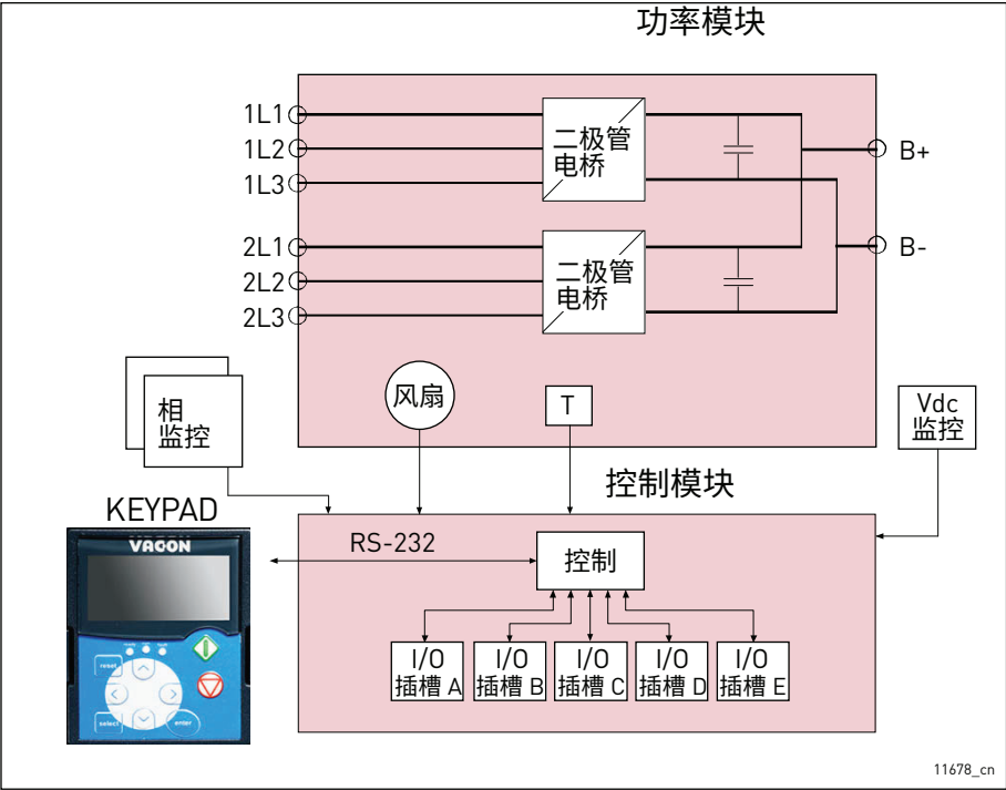
图 119. 非再生前端模块示意图
