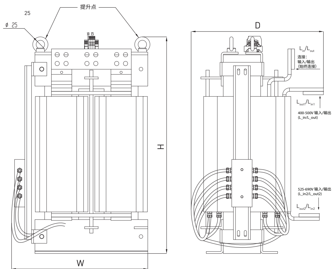
图 106. VACON® RLC 滤波器的 L_{afe} 电抗器示例
