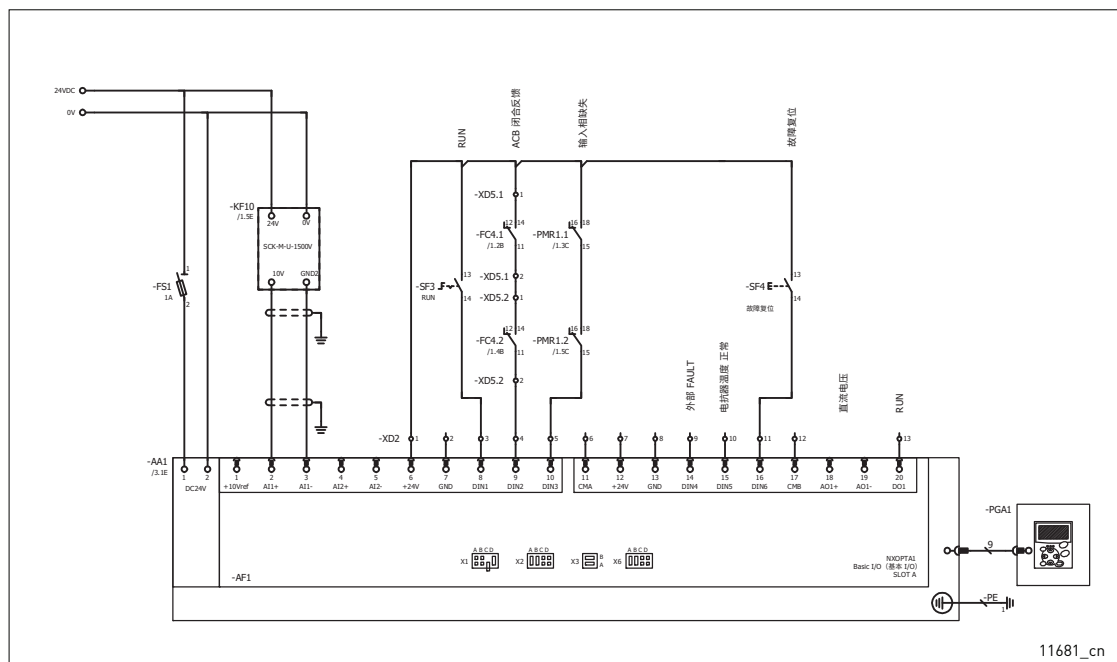
图 116. 控制装置接线图，OPTA1。
