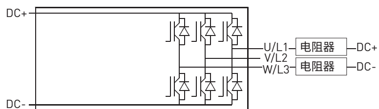
图 124. 制动斩波器单元拓扑
