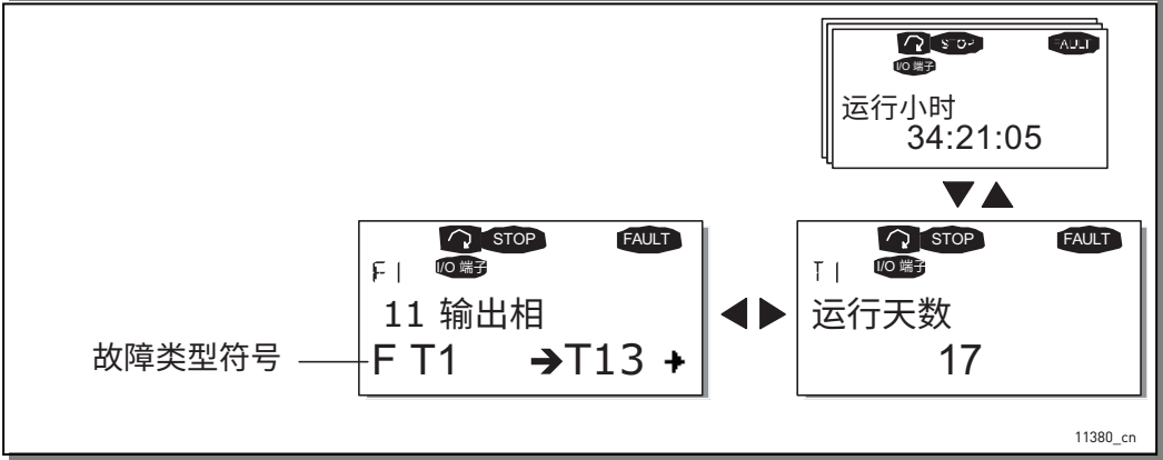
图 83. 故障显示
