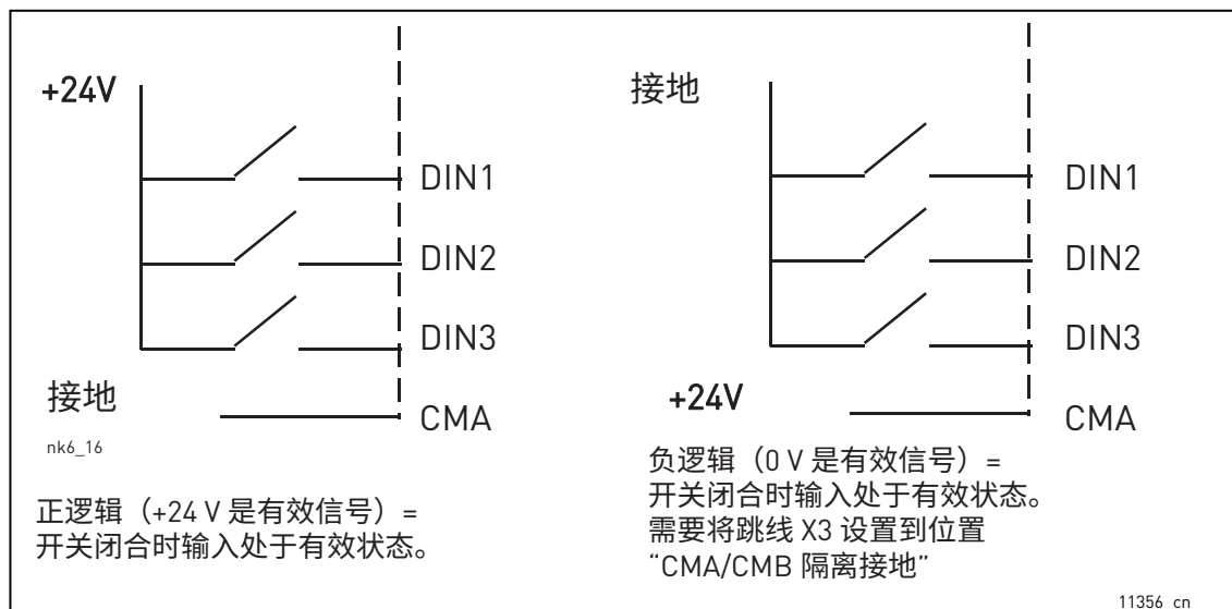
图 64. 正 / 负逻辑
