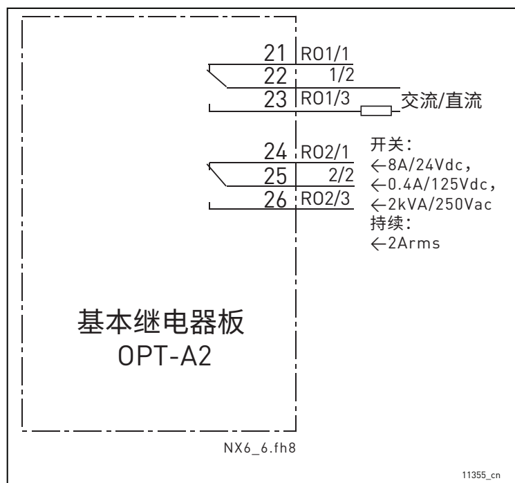
图 62. 基本继电器板 (OPT-A2) 的一般接线图
