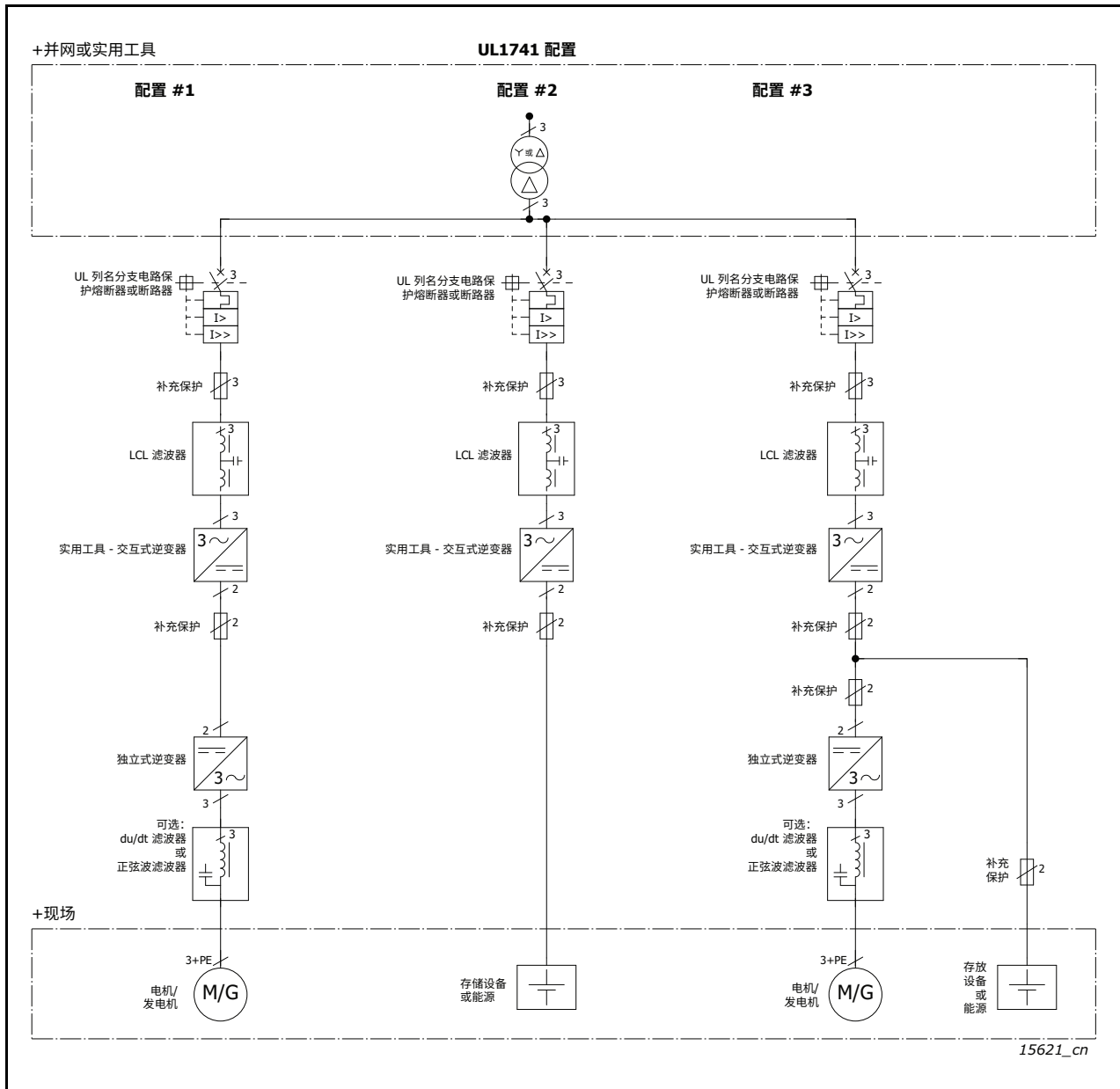
图 131. UL1741 的并网变流器配置的单线路图
