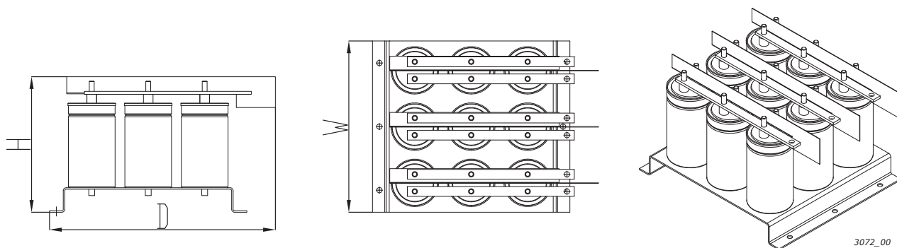
图 107. VACON® RLC 滤波器的电容器组 ( C_{bank} ) 示例
