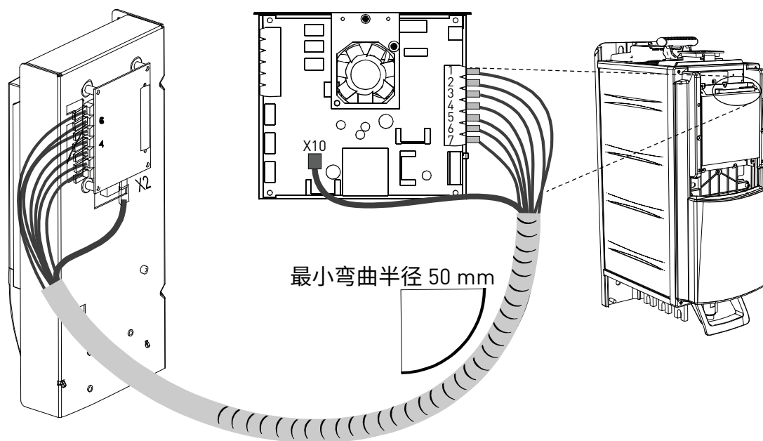
图 73. 将电源和控制电缆连接到控制单元，Ch6x
