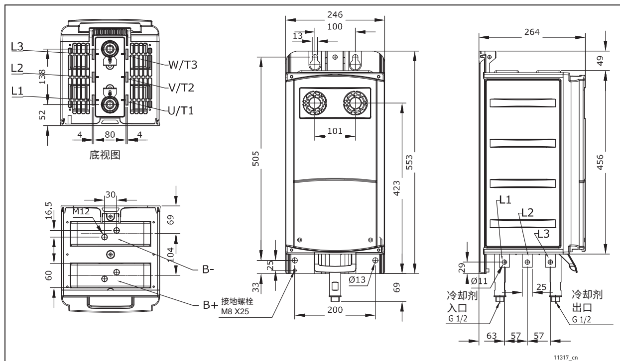
图 10. VACON® NX 水冷式变频器尺寸, CH5
