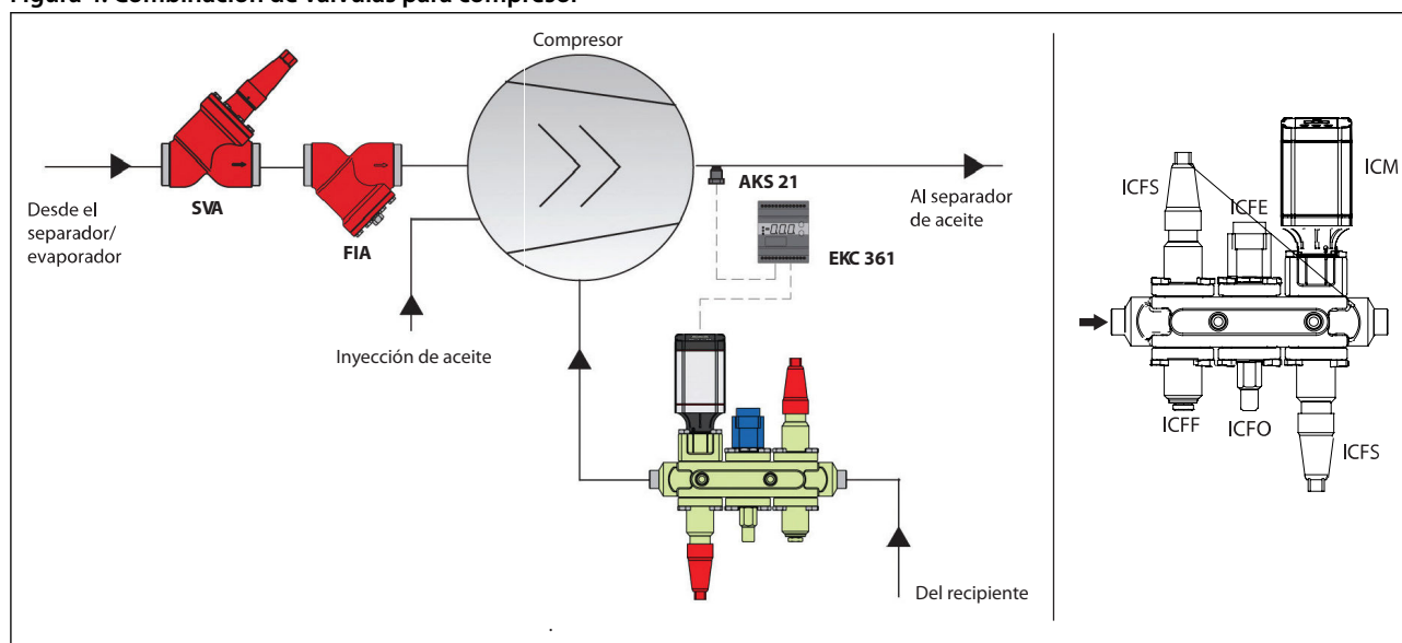
Figura 4: Combinación de válvulas para compresor
