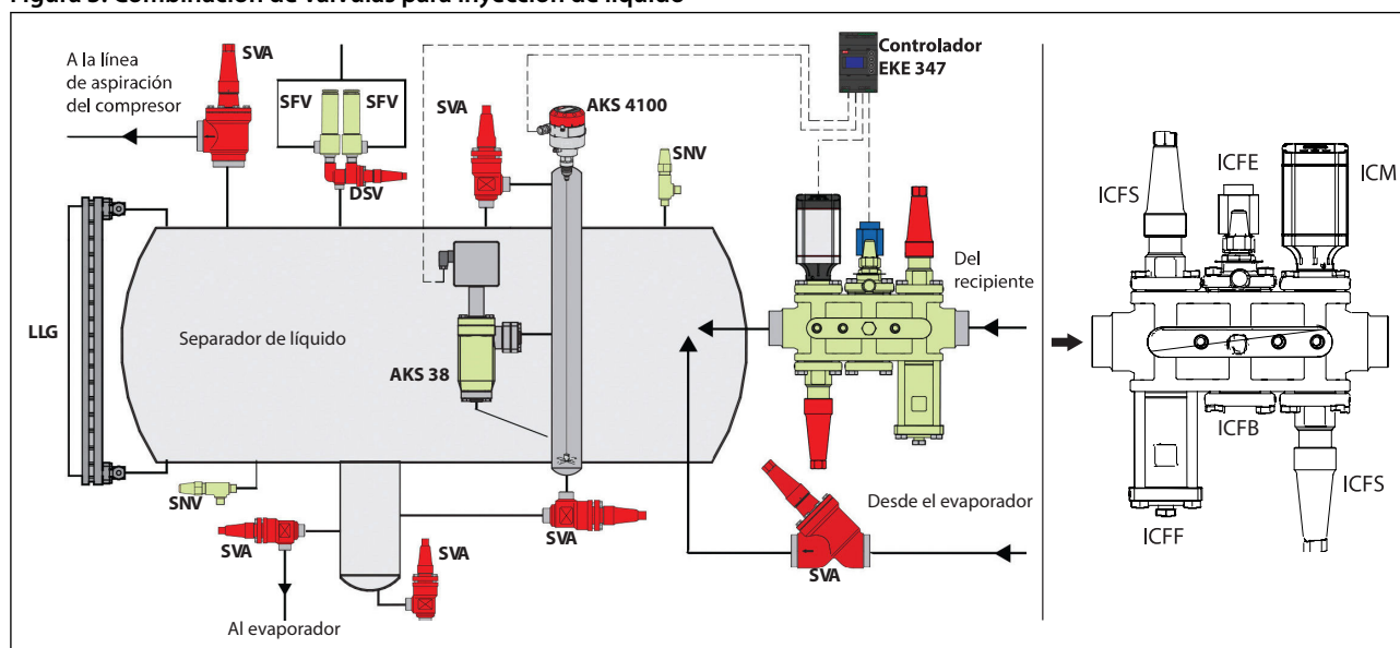
Figura 3: Combinación de válvulas para inyección de líquido
