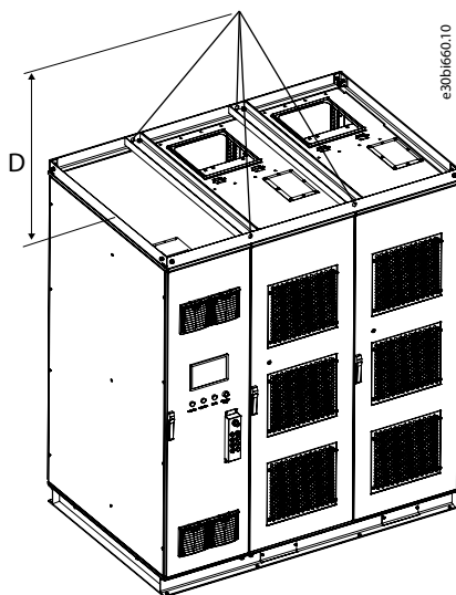
Illusztráció 33: A teljesítménycella-szekrény emelési pontjai
