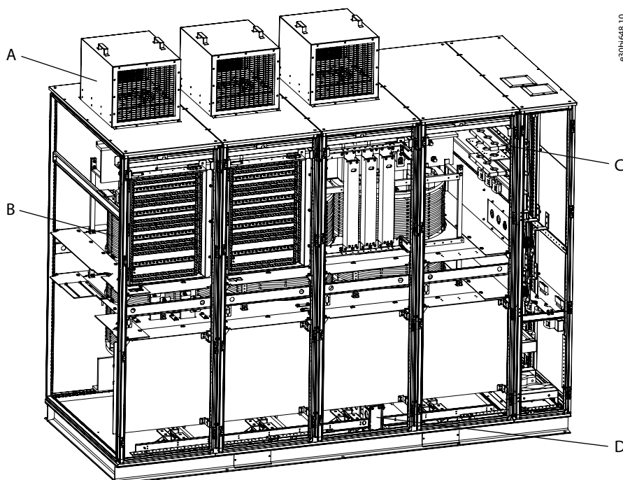
Illusztráció 11: Transzformátorszekrény a VACON® 1000 line-up rendszereiben
