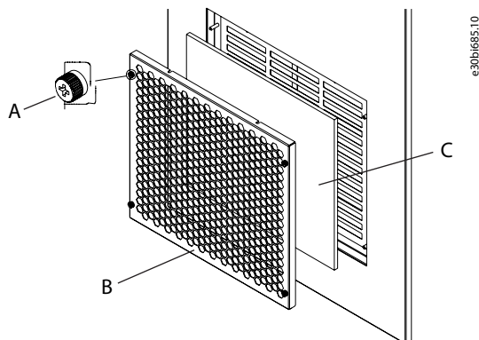
Illusztráció 72: Légszűrő cseréje
