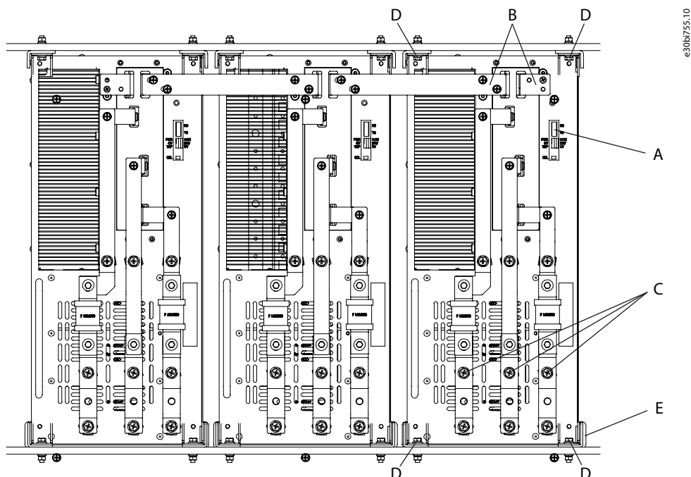
Illusztráció 81: Teljesítménycella cseréje
