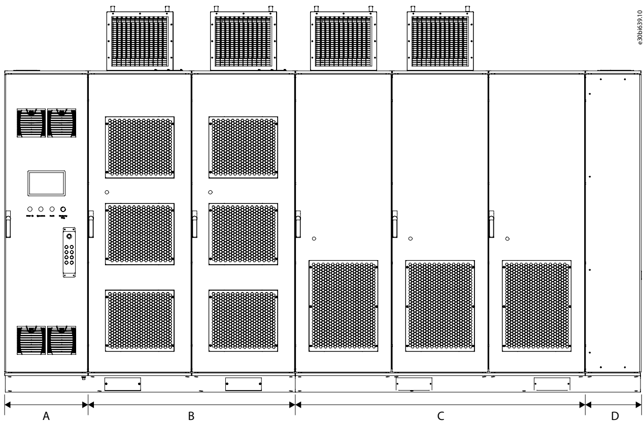
Illusztráció 2: Line-up rendszer felépítése
