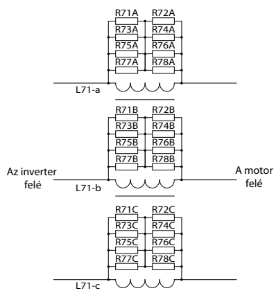
Illusztráció 15: A kimeneti szűrőszekrény kapcsolási rajza
