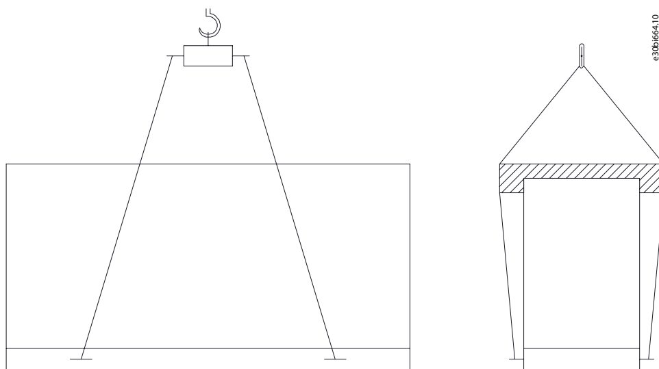
Illusztráció 32: Egy fadarabbal szétfeszített emelőkötelek
