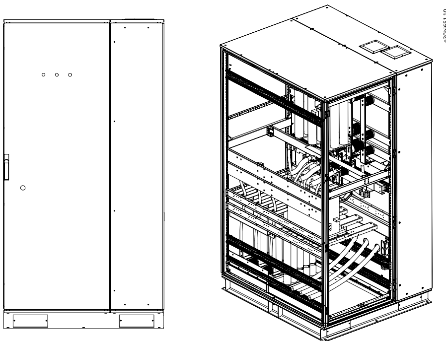
Illusztráció 13: Indítószekrény
