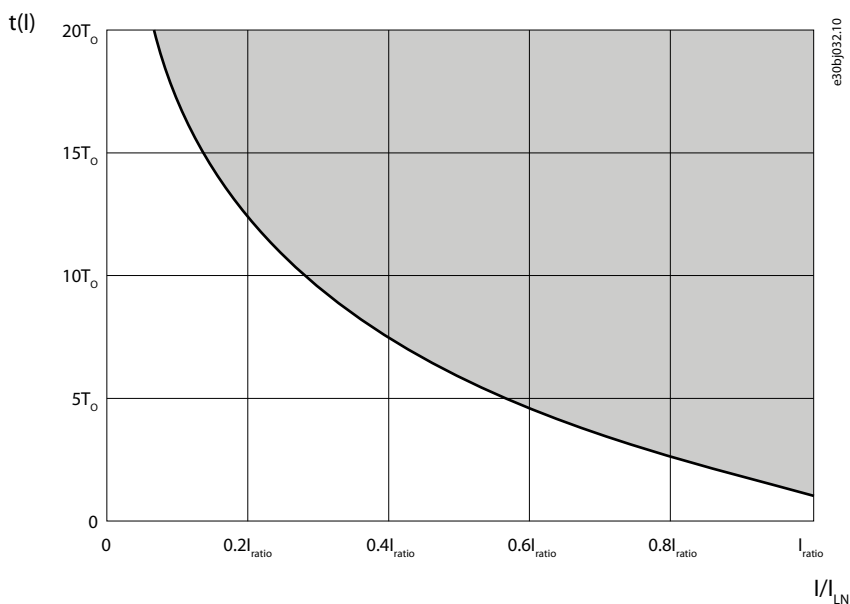
Illusztráció 14: A túláramvédelem beállítási területe
