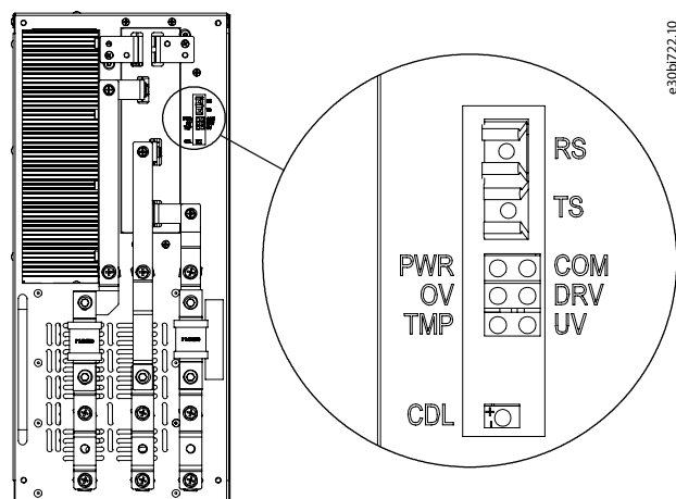
Illusztráció 80: A teljesítménycella jelzőfényének helye
