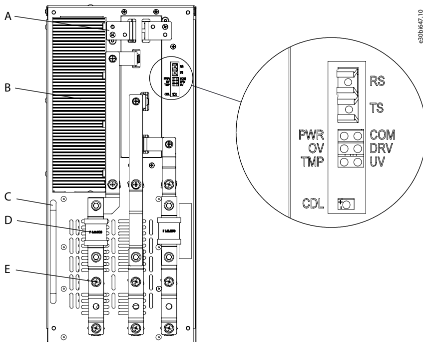
Illusztráció 9: Teljesítménycella
