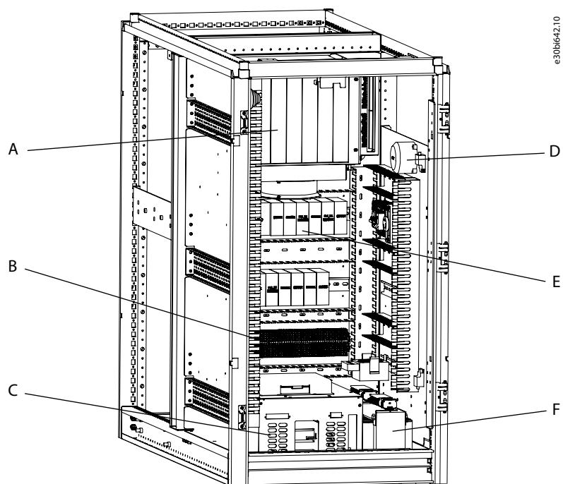
Illusztráció 3: Vezérlőszekrény a VACON® 1000 önálló rendszereiben
