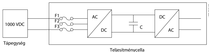
Illusztráció 84: Az DC-tápegység vezetékezési rajza
