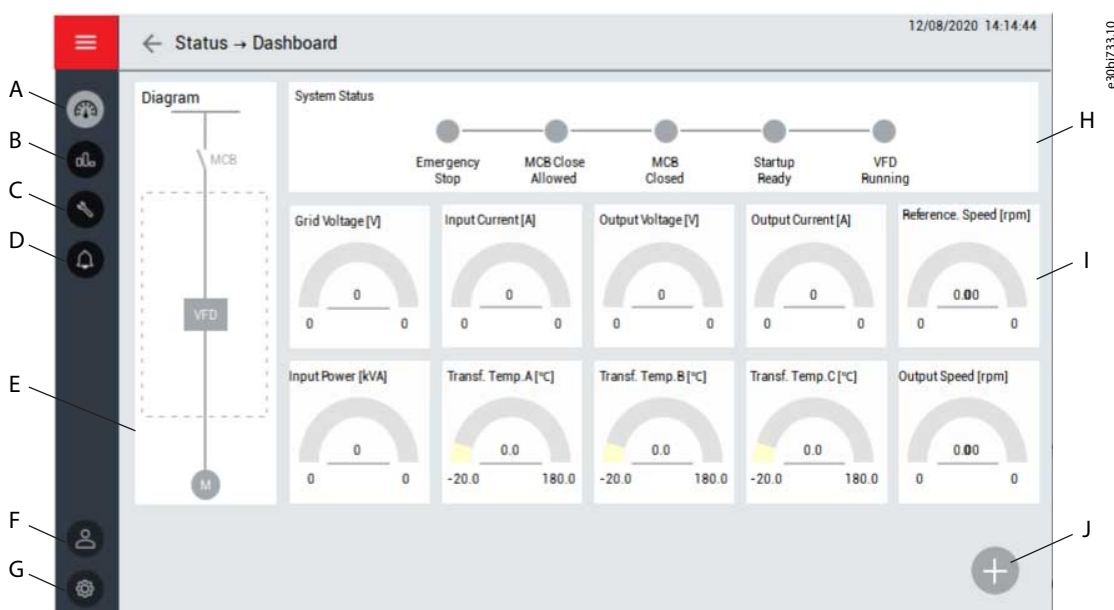
Illusztráció 55: A HMI kezdőlapja
