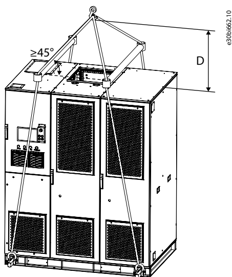
Illusztráció 30: Az önálló szekrények emelése
