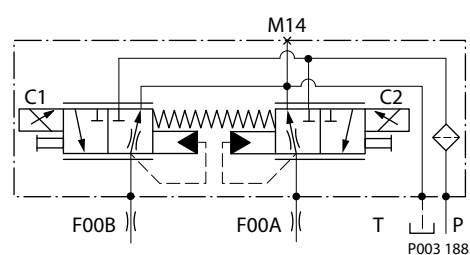
NFPE 回路図
