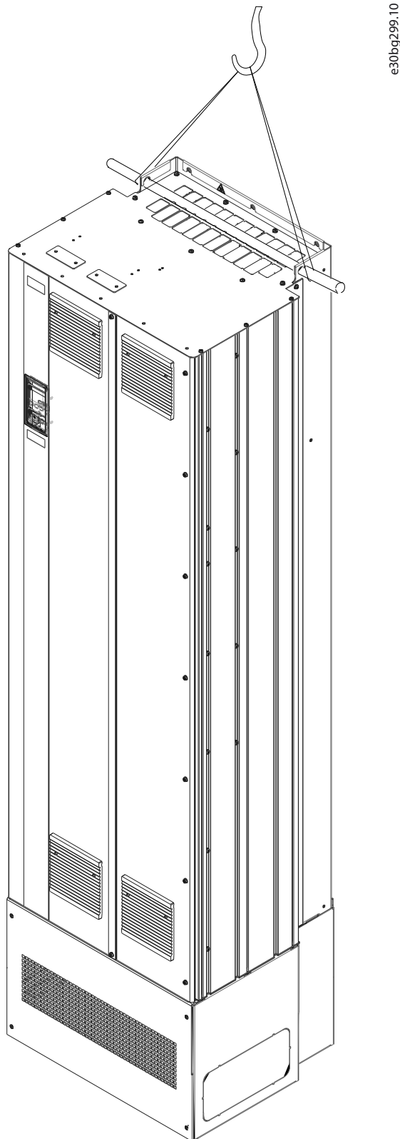
Ilustración 39: Montaje en pedestal
