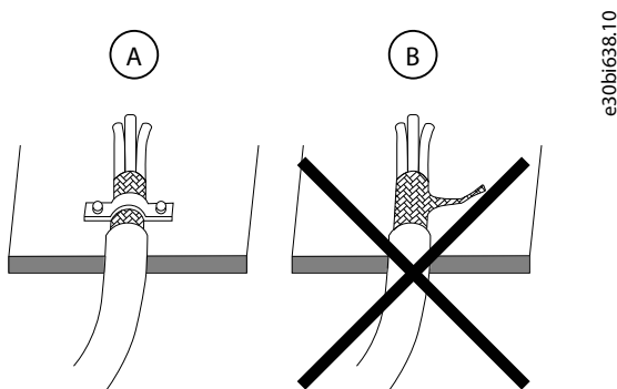
Ilustración 49: Instalación del apantallamiento de cables
