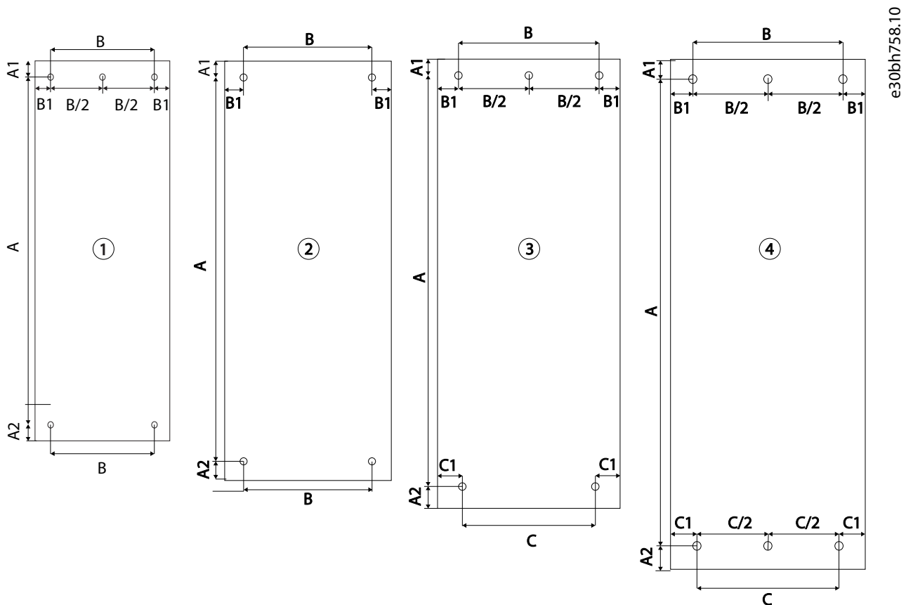
Ilustración 41: Patrones de perforación para bastidores FA02-FA12
