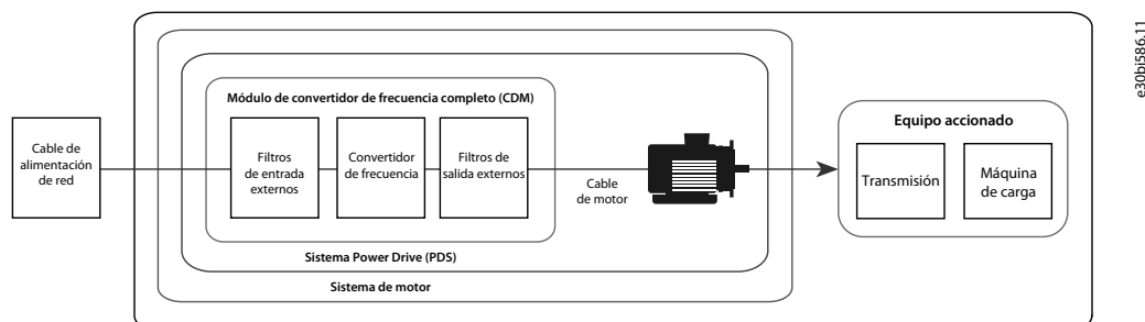
Ilustración 2: Diseño del accionamiento eléctrico de potencia
