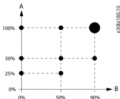
Ilustración 1: Punto de funcionamiento conforme a IEC 61800-9-2
