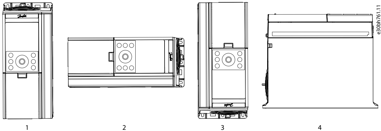
Ilustración 40: Direcciones de montaje de los convertidores
