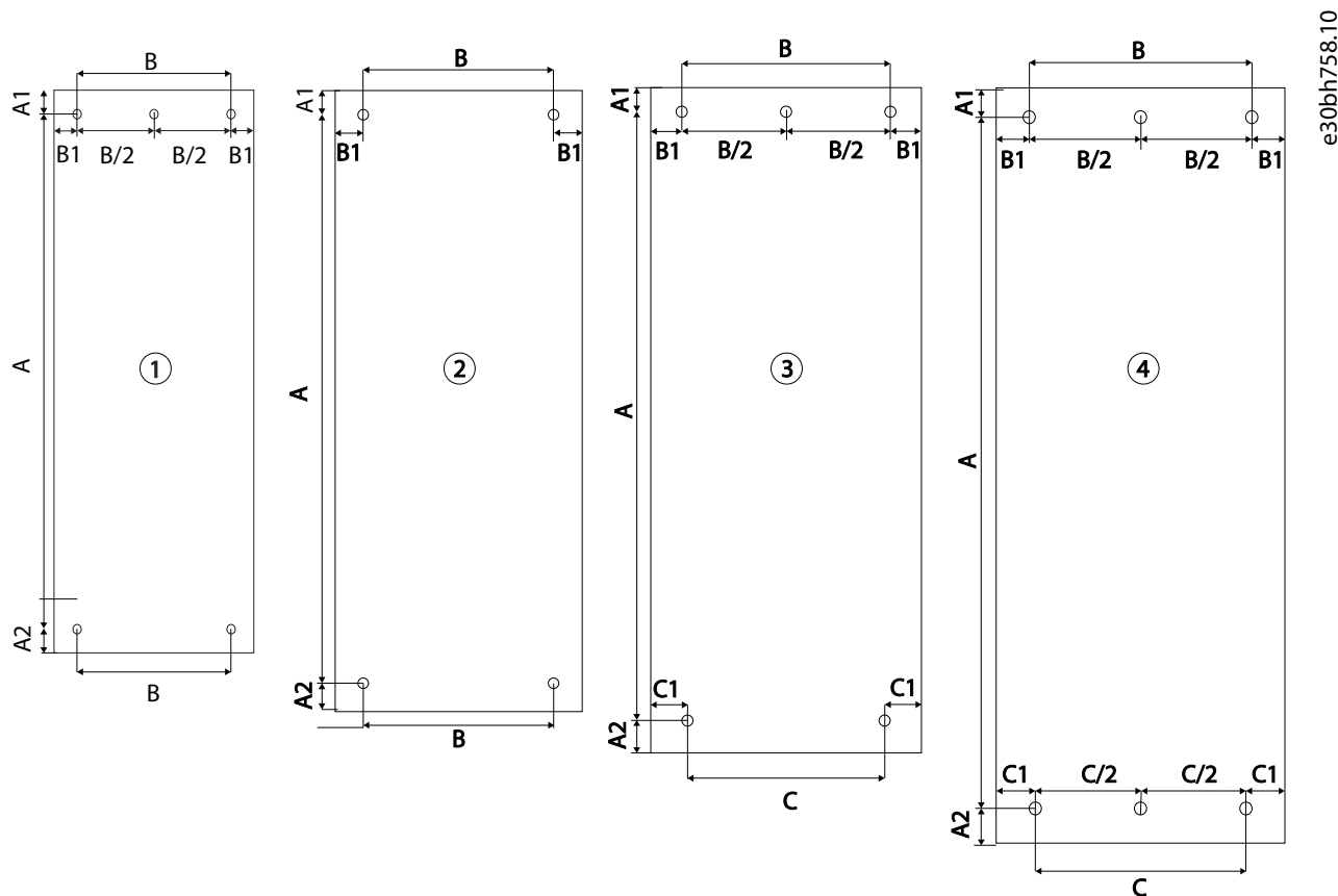
Illustration 41: Schémas de perçage pour les châssis FA02-FA12
