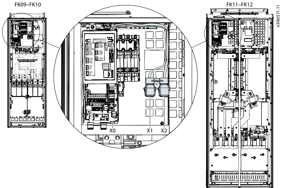
Illustration 56: Emplacements des ports de communication X0, X1 et X2 dans les châssis FK09-FK12
