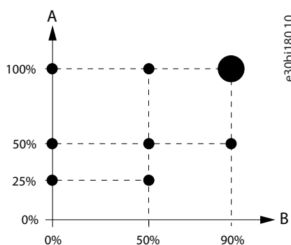
Illustration 1: Point de fonctionnement selon la norme CEI 61800-9-2
