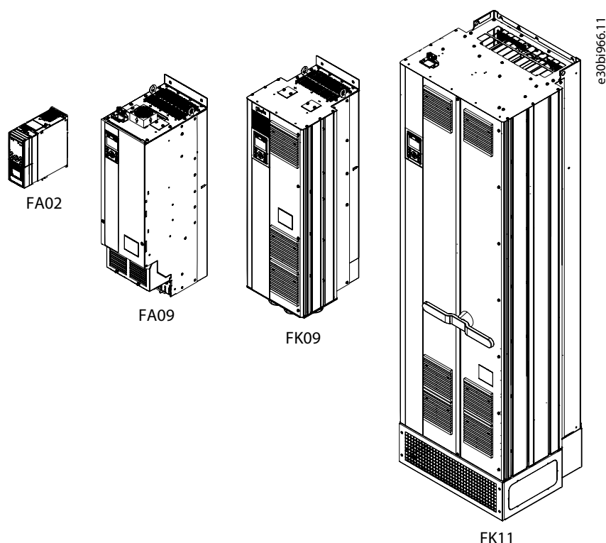
Illustration 3: Offre de châssis dans la gamme iC7-Automation
