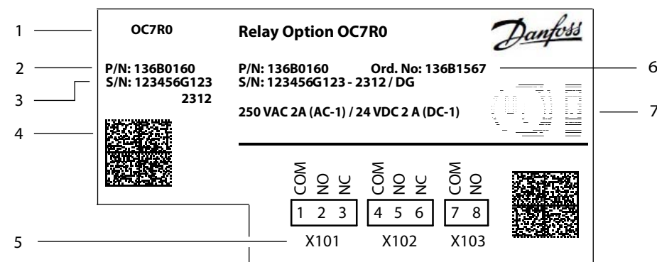
Illustration 25: Exemple d'étiquette de produit sur une extension fonctionnelle
