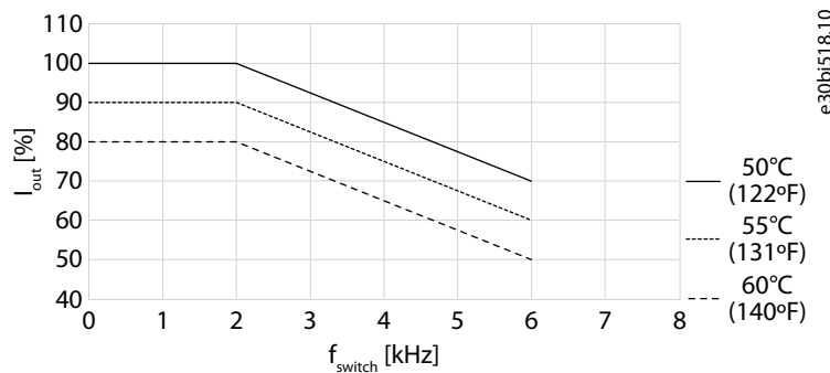
Illustration 36: Déclassement du courant de sortie par rapport à la fréquence de commutation pour Fx11-Fx12 avec surcharge élevée (HO1)
