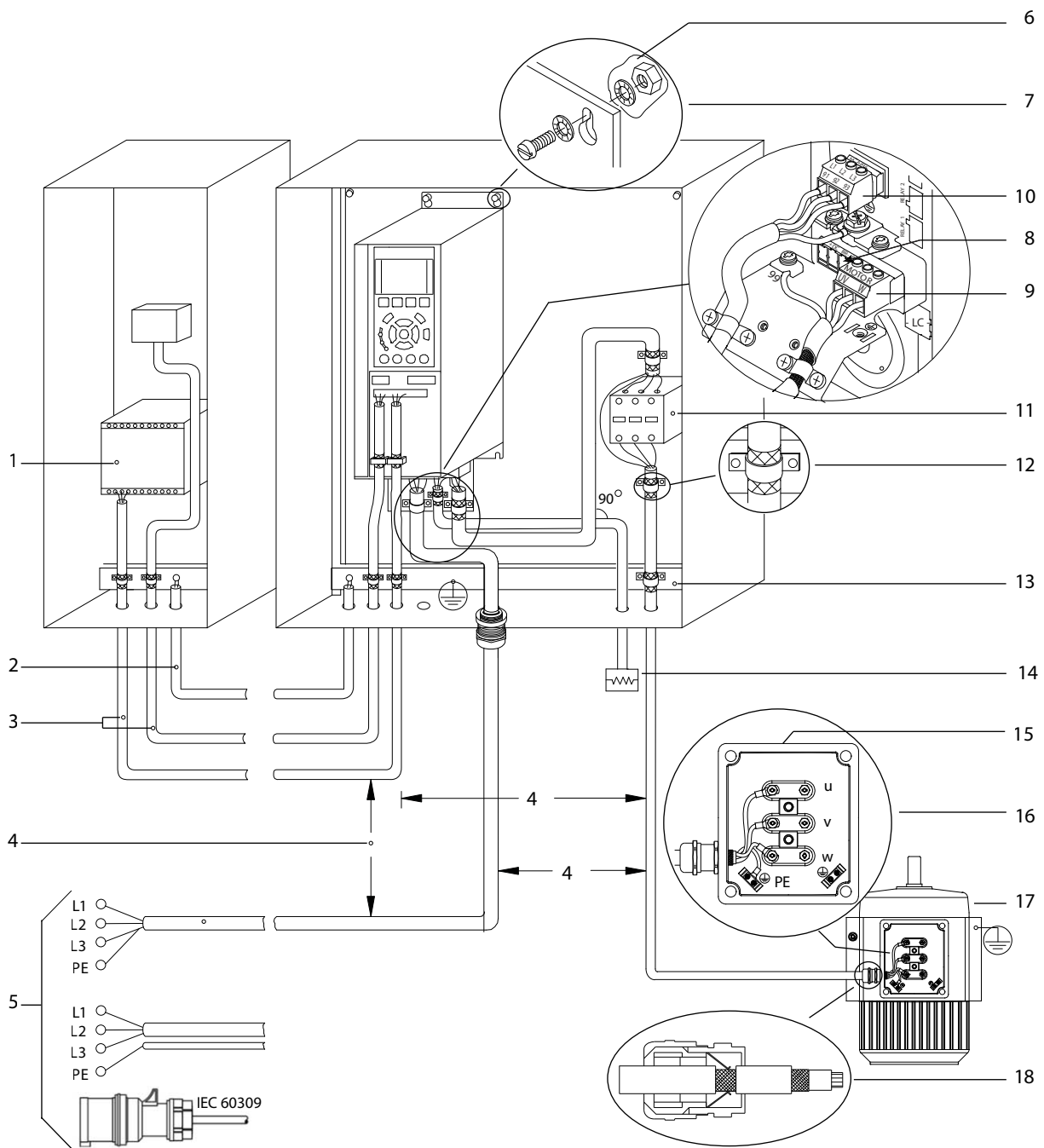
Illustration 48: Exemple d'installation conforme aux exigences CEM
