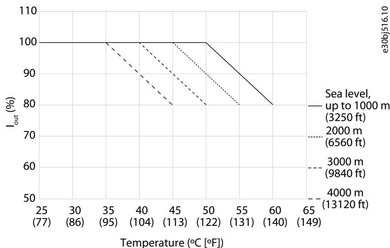
Illustration 29: Déclassement du courant de sortie en fonction de l'altitude et de la température ambiante (châssis Fx09-Fx12, surcharge élevée)
