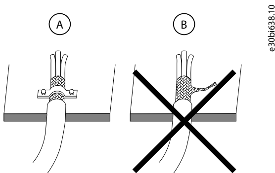
Illustration 49: Installation du blindage de câble
