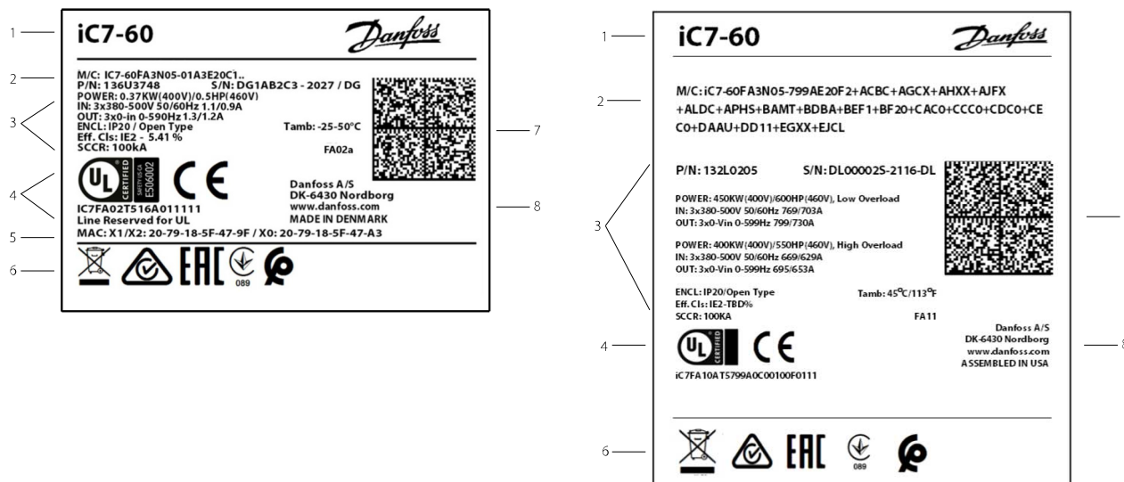
Illustration 23: Étiquettes de produit pour Fx02-Fx08 (gauche) et Fx09-Fx12 (droite)
