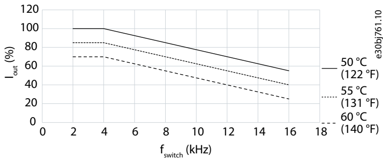
Illustration 31: Déclassement du courant de sortie par rapport à la fréquence de commutation (FA05) en cas de surcharge faible (LO) et élevée (HO1)
