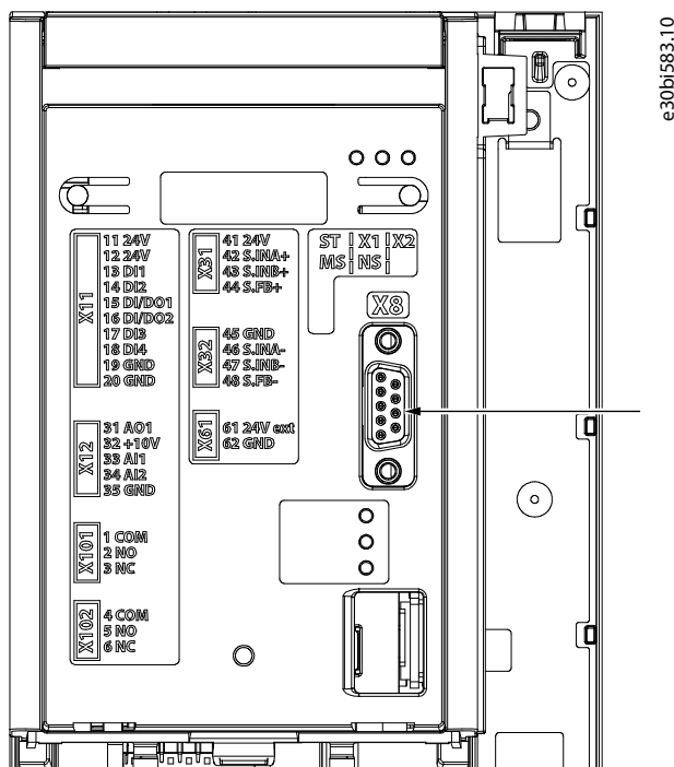
Illustration 57: Emplacement du connecteur X8
