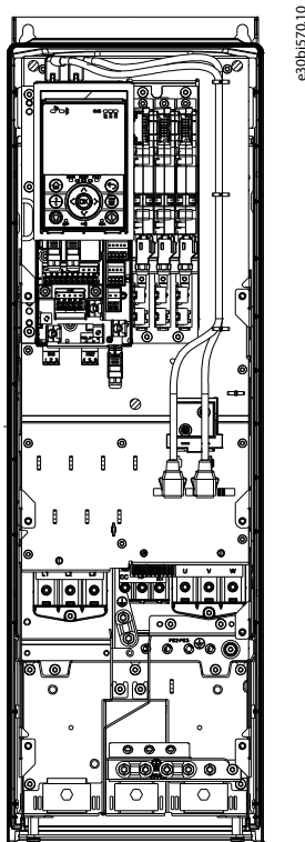
Illustration 58: Chemin des câbles pour châssis FK06-FK08
