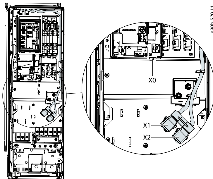
Illustration 55: Emplacements des ports de communication X0, X1 et X2 dans les châssis FK06-FK08
