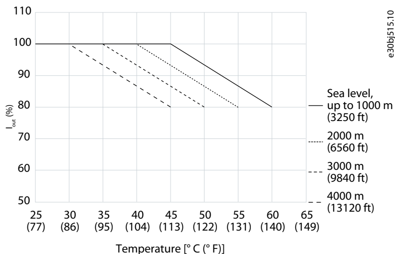
Illustration 28: Déclassement du courant de sortie en fonction de l'altitude et de la température ambiante (châssis Fx09-Fx12, surcharge faible)
