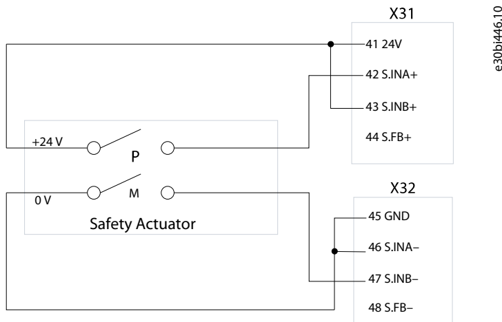
Illustration 62: Exemple de raccordement STO utilisant différentes polarités
