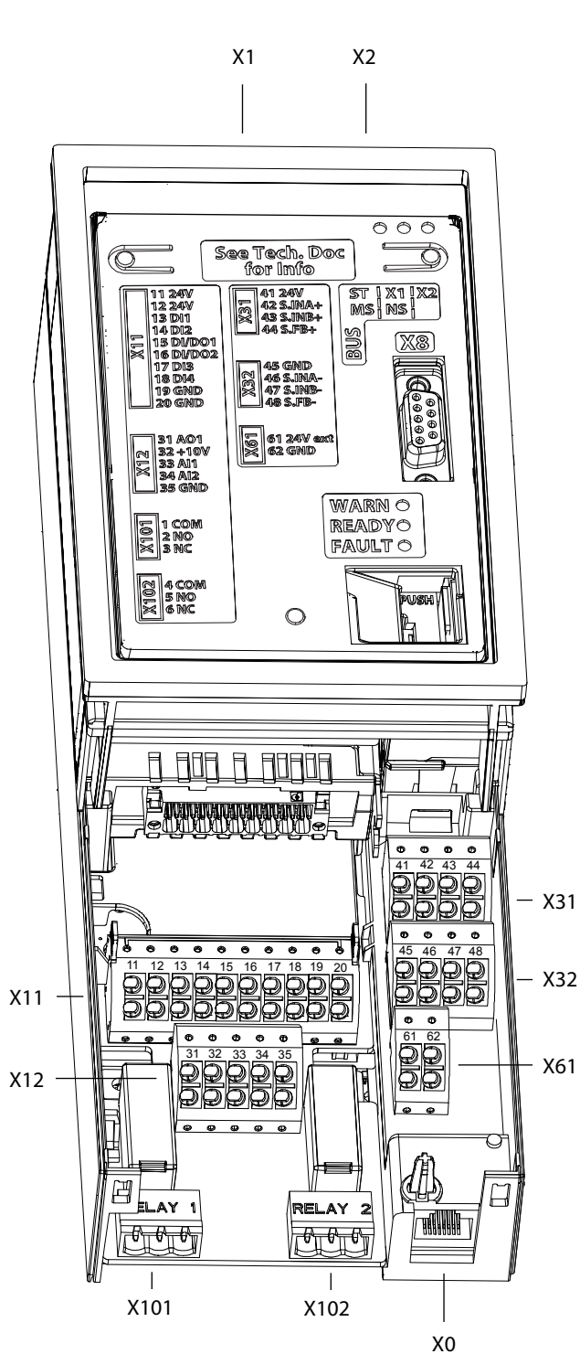
Illustration 51: Emplacement des connexions sur la carte de commande sans option d'extension fonctionnelle
