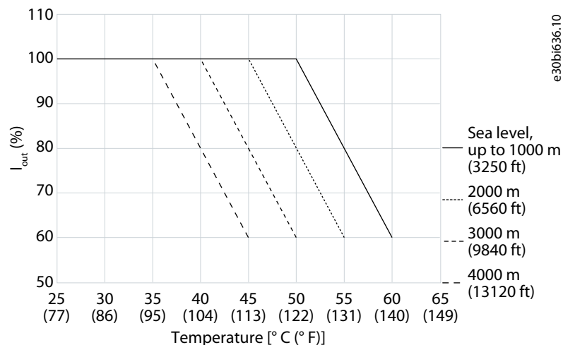
Illustration 27: Déclassement du courant de sortie en fonction de l'altitude et de la température ambiante (châssis FA02-FA08)
