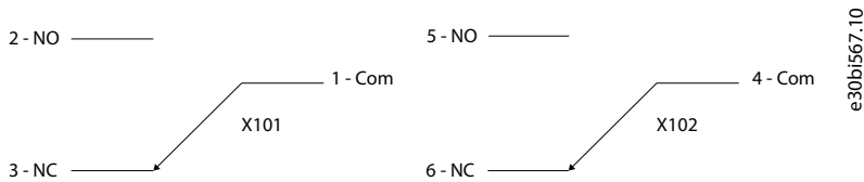
Illustration 52: Fonctionnalité des relais X101 et X102
