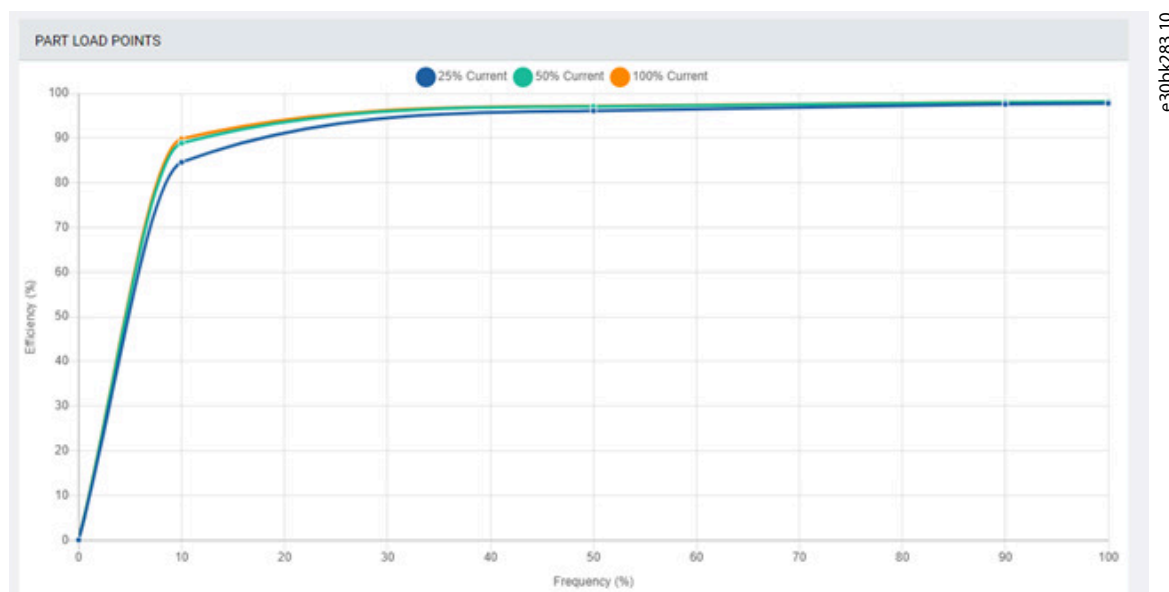
Illustration 9: Exemple de données MyDrive® ecoSmart™
