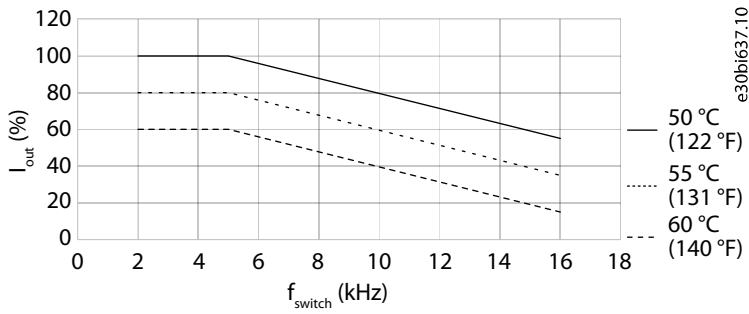
Illustration 30: Déclassement du courant de sortie par rapport à la fréquence de commutation (FA02-FA04) en cas de surcharge faible (LO) et élevée (HO1)
