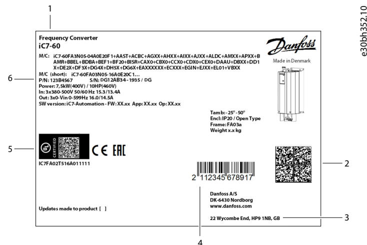
Illustration 24: Exemple d'étiquette d'emballage
