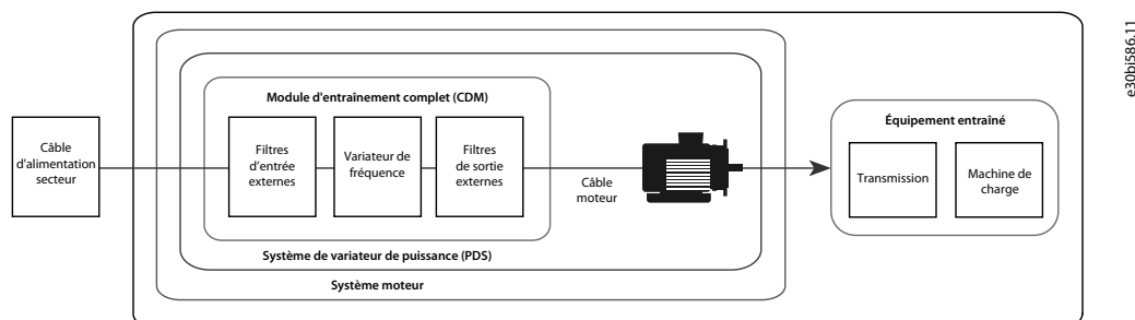
Illustration 2: Conception du système de variateur
