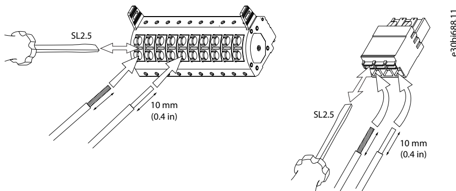
Illustration 59: Insertion des fils dans le connecteur
