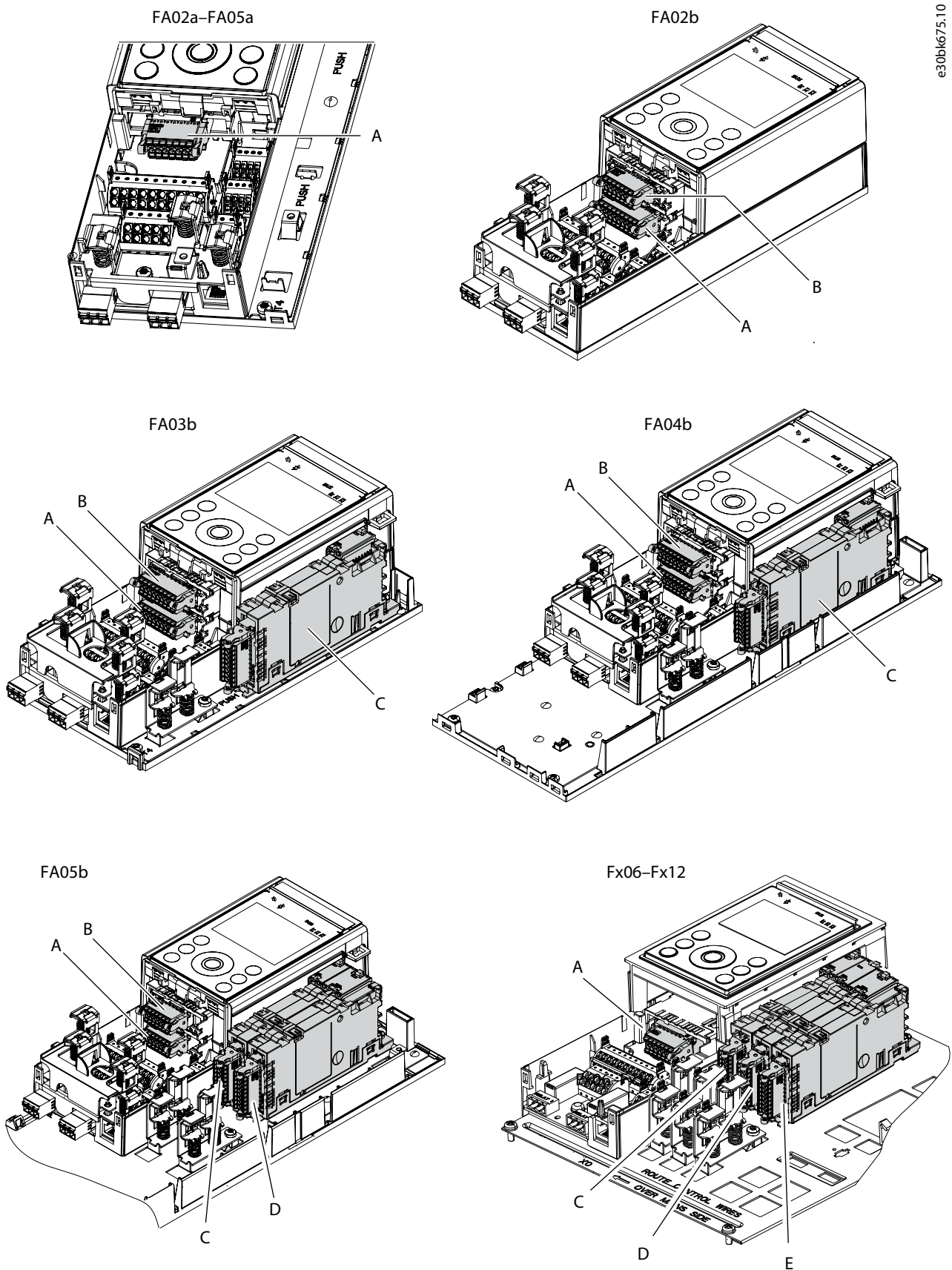
Illustration 7: Emplacements d'option dans les variateurs de fréquence iC7-Automation
