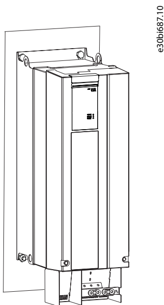
Illustration 37: Montage sur un mur ou dans une armoire
