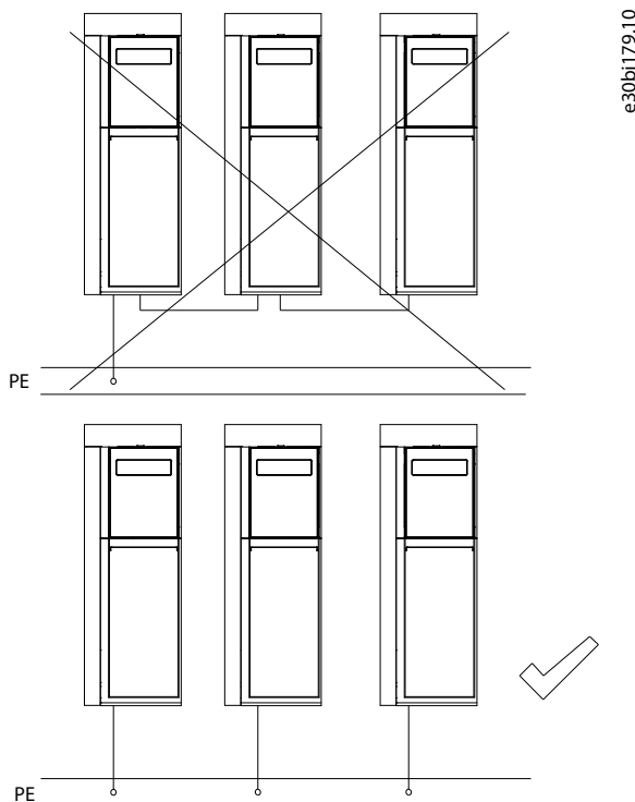
Illustration 50: Principe de mise à la terre
