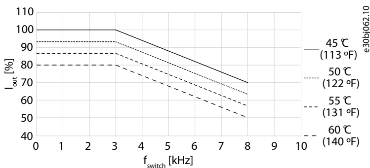
Illustration 33: Déclassement du courant de sortie par rapport à la fréquence de commutation pour Fx09-Fx10 avec surcharge faible (LO)
