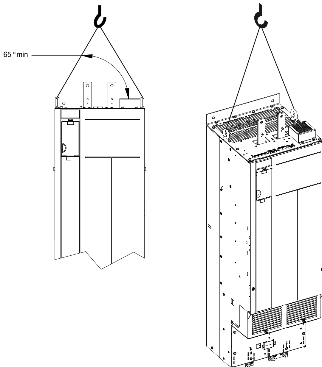
Illustration 42: Levage des châssis Fx06-Fx10 à l'aide d'anneaux de levage
