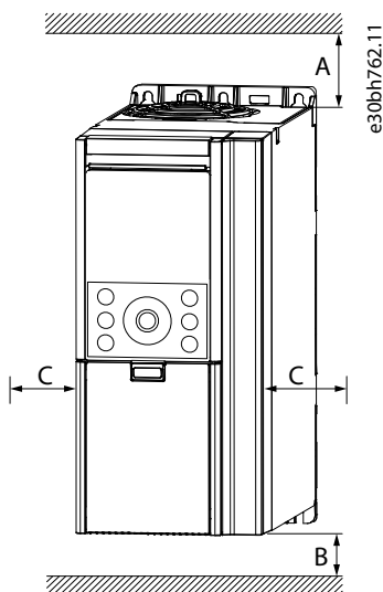
Illustration 44: Dégagement pour le refroidissement
