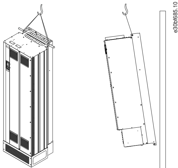
Illustration 43: Levage des châssis Fx11-Fx12 à l'aide d'une barre de levage
