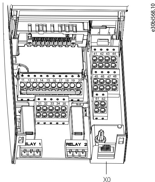
Illustration 53: Emplacement du port X0 sur la carte de commande
