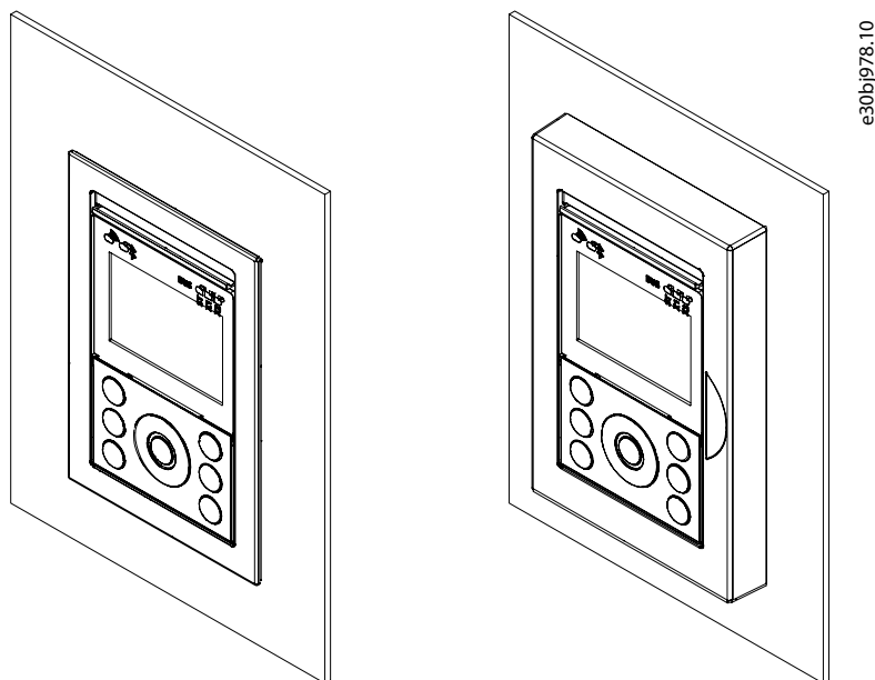
Illustration 8: Panneau de commande monté dans le kit de montage aligné (gauche) et kit de montage panneau sur porte (droite)
