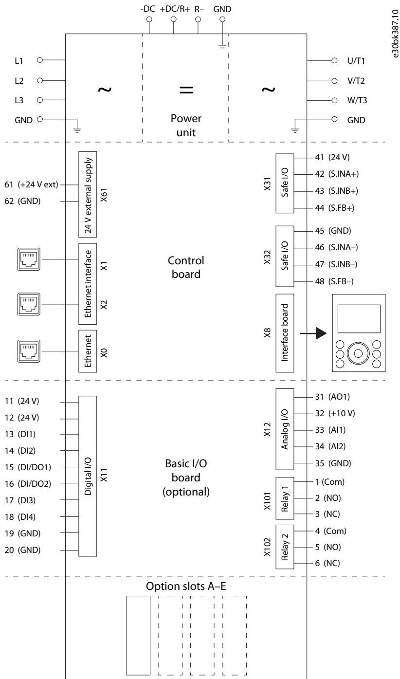
Illustration 46: Schéma de câblage des variateurs de fréquence avec carte de commande Ethernet
