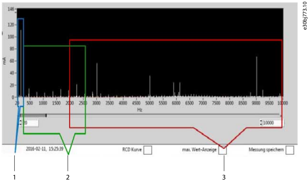
Illustration 47: Exemple de mesure FFT
