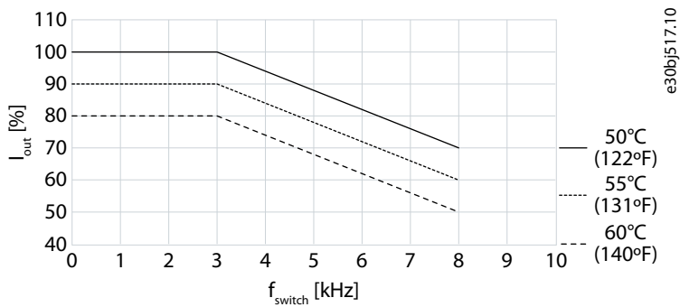
Illustration 35: Déclassement du courant de sortie par rapport à la fréquence de commutation pour Fx09-Fx10 avec surcharge élevée (HO1)
