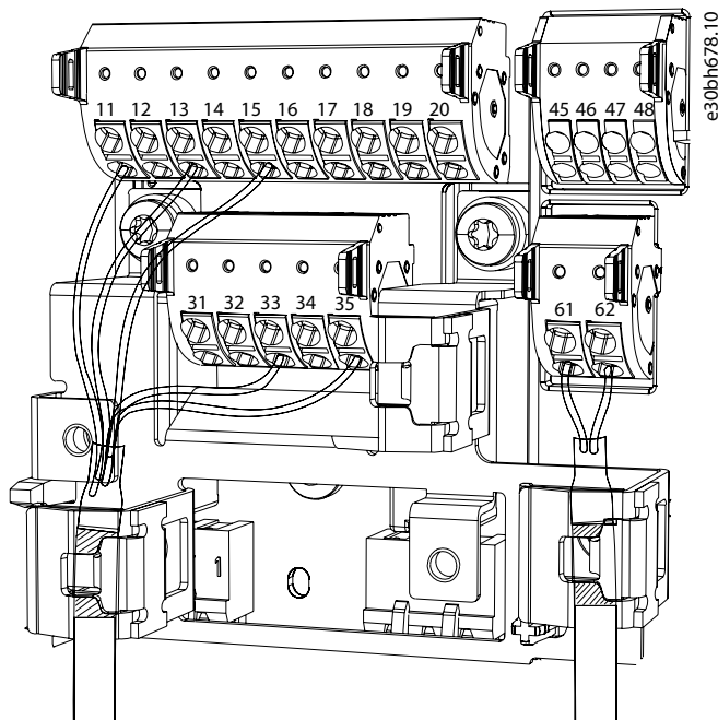
Illustration 60: Raccordement correct du blindage de câble
