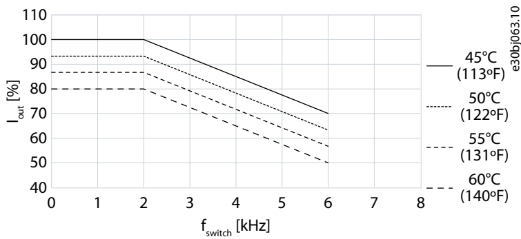
Illustration 34: Déclassement du courant de sortie par rapport à la fréquence de commutation pour Fx11-Fx12 avec surcharge faible (LO)
