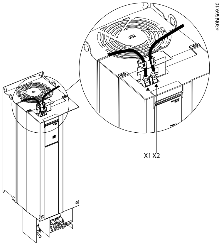
Illustration 54: Emplacement de l'interface de communication, X1/X2 dans les châssis FA02-FA12 (avec la plaque CEM en option)
