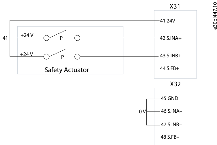
Illustration 61: Exemple de raccordement STO utilisant les mêmes polarités (canal A et canal B = 24 V)
