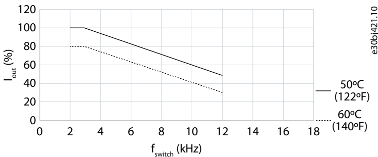
Illustration 32: Déclassement du courant de sortie par rapport à la fréquence de commutation (Fx06-Fx07) en cas de surcharge faible (LO) et élevée (HO1)
