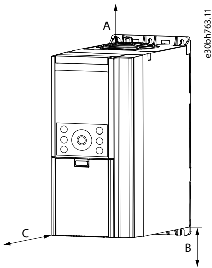
Illustration 45: Dégagement recommandé pour l'accès pour entretien
