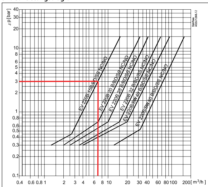
Bild 5: Leistungsdiagramm
