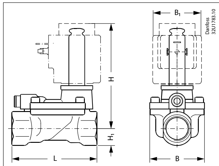
Bild 7: Maße
