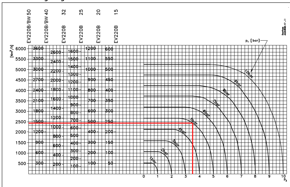
Bild 6: Leistungsdiagramm
