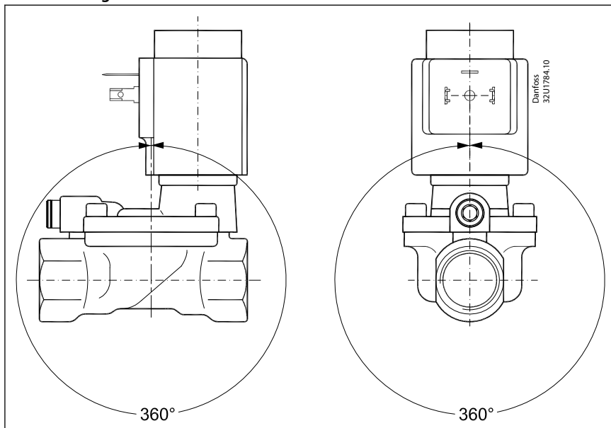
Bild 8: Montagewinkel
