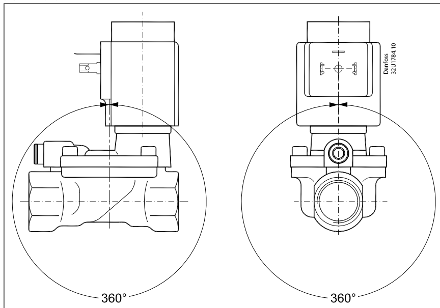
图 8: 安装角度
