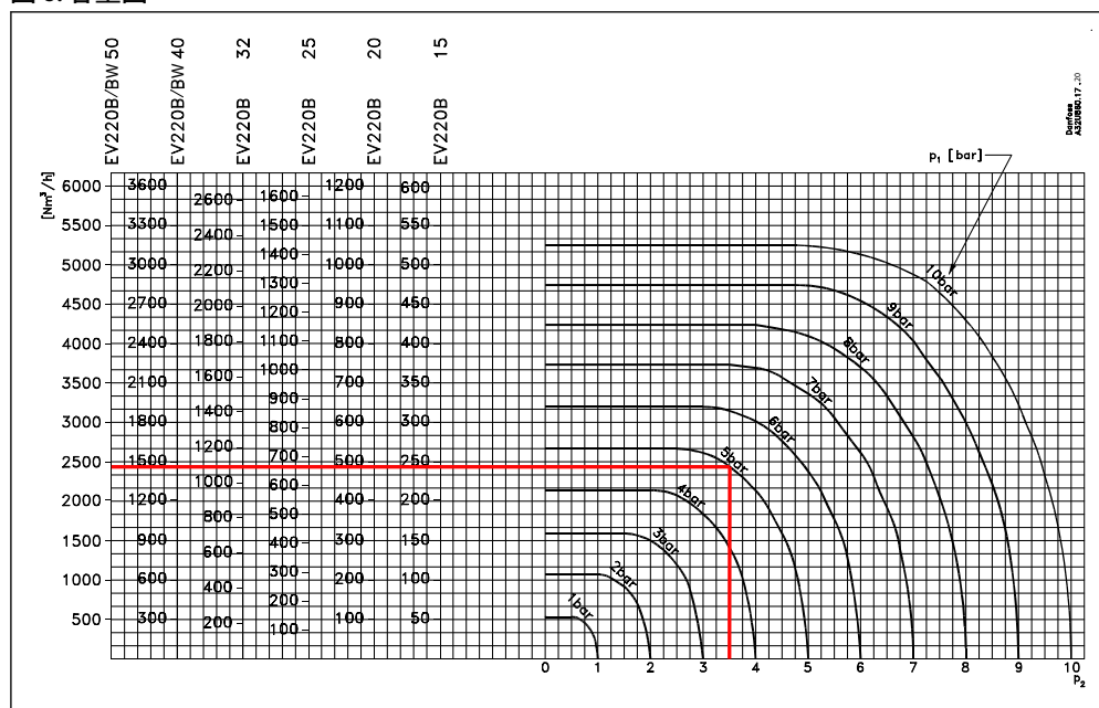
图 6: 容量图
