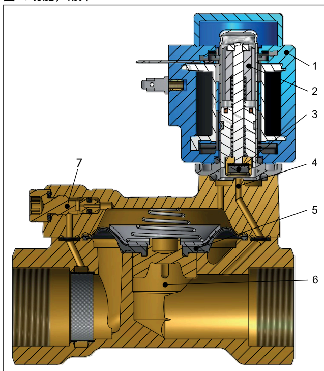
图 2: 功能，常开
