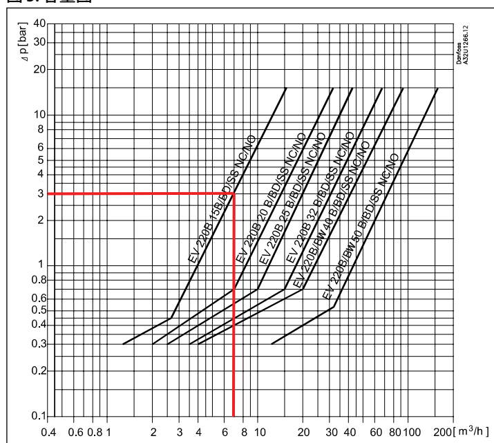
图 5: 容量图
