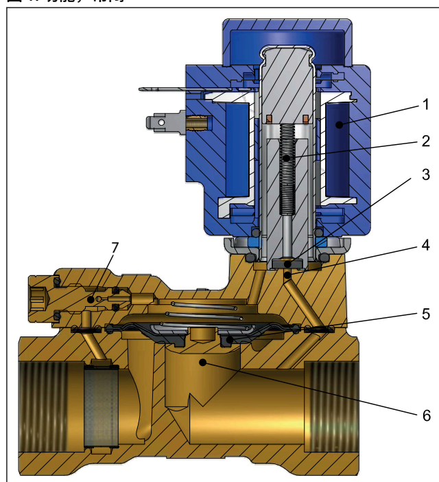
图 1: 功能，常闭
