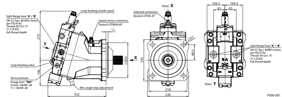
Abbildung 2: DIN ISO 3019/2, mit elektrischer Proportionalverstellung (Stromlos = min. Schluckvolumen)
