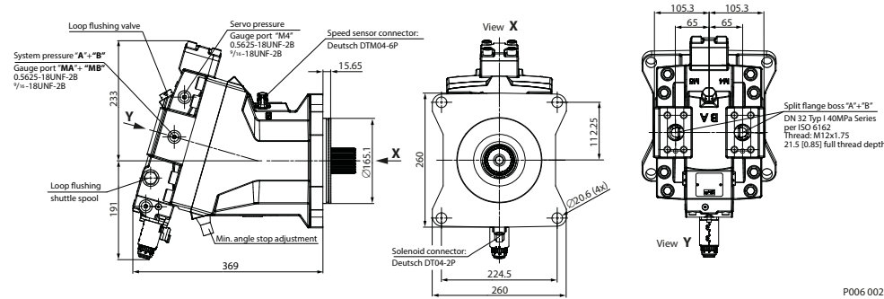
Abbildung 2: DIN ISO 3019/2, mit elektrischer Proportionalverstellung (Stromlos = min. Schluckvolumen)
