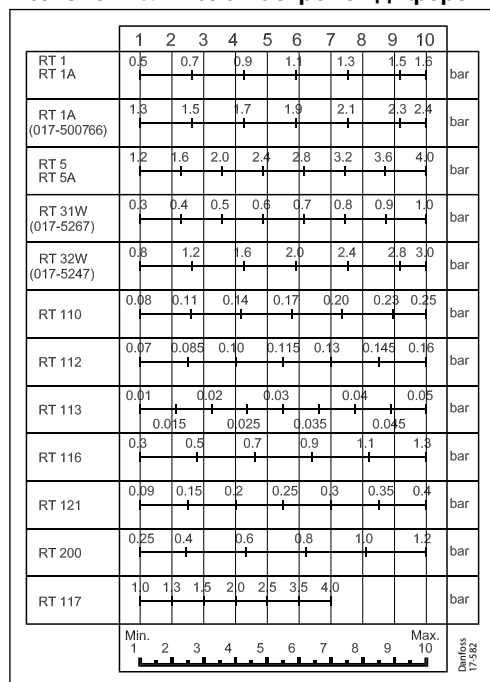
Малюнок 26: Шкала настройок диференціалу
