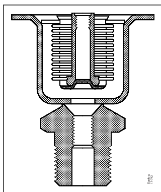
Мал 4: Поперечний переріз реле RT 32W
