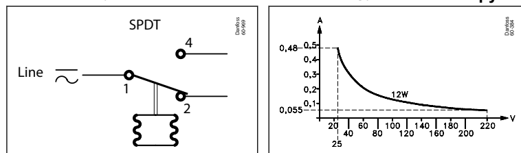
Малюнок 22: Система контактів Малюнок 23: Постійний струм
