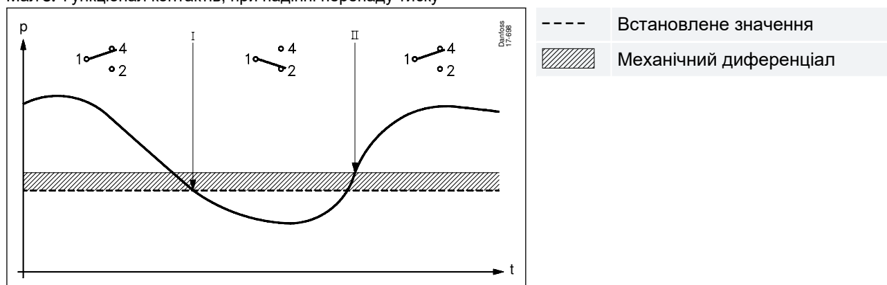
Мал 8: Функціонал контактів, при падінні перепаду тиску
