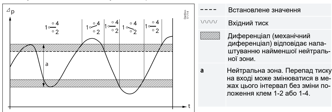
Мал 9: Функціонал контактів, налаштування нейтральної зони
