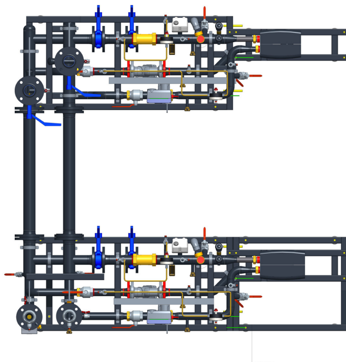
Raccordement en parallèle **
