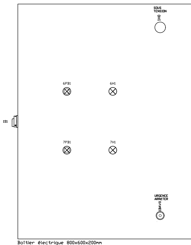
Boîtier électrique 800x600x200mm
