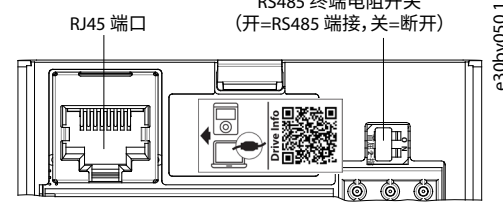
图 4: RJ45 端口和 RS485 端接开关
