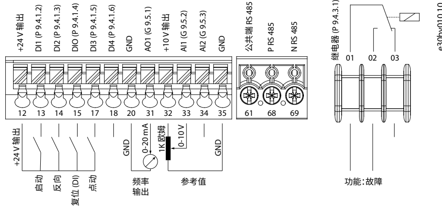
图 3: 默认设置为 PNP 配置 (速度控制模式) 的控制端子概述
