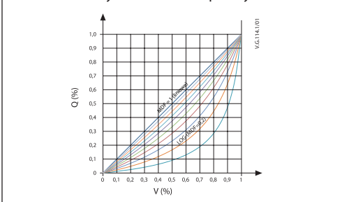
AV:4/32772 Krzywa wartości współczynnika alfa
