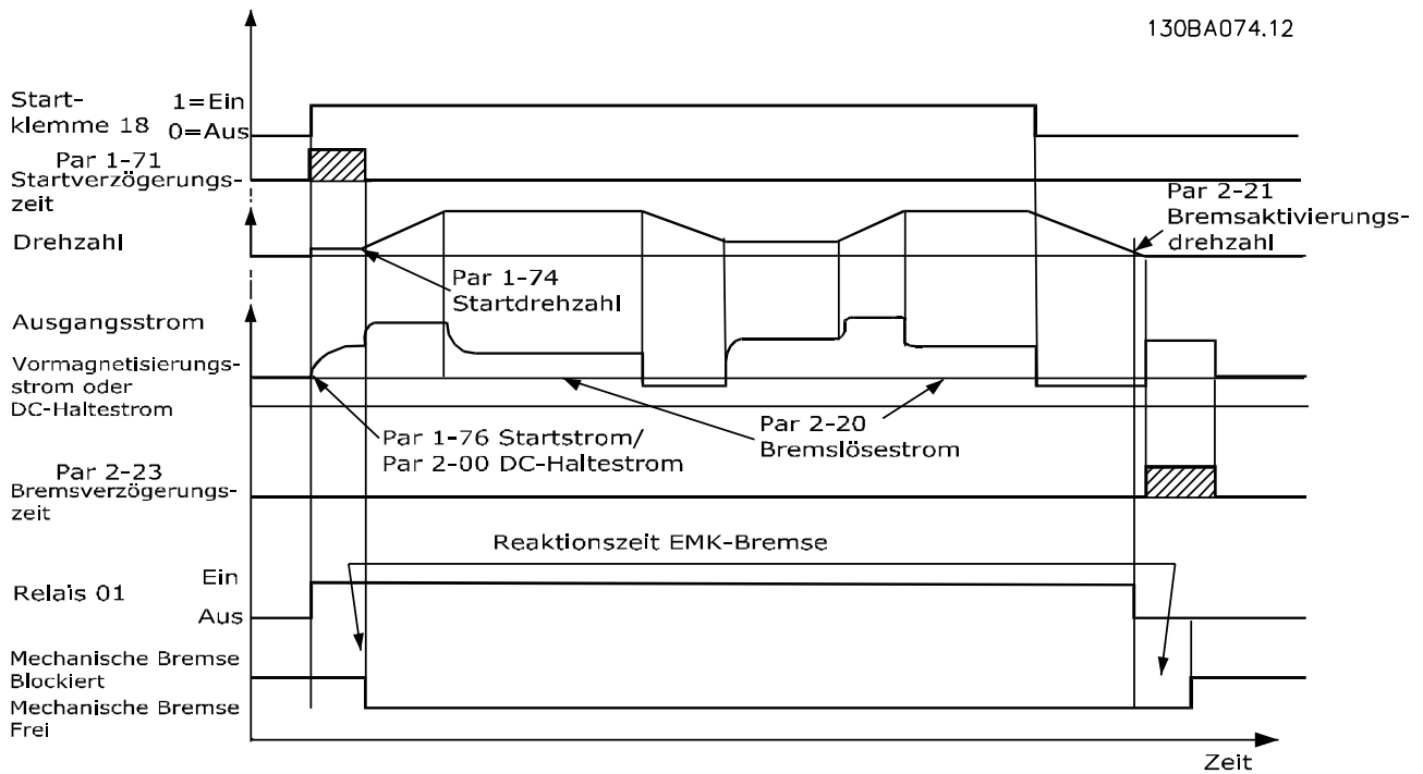
Abbildung 4.2 Mechanische Bremse
