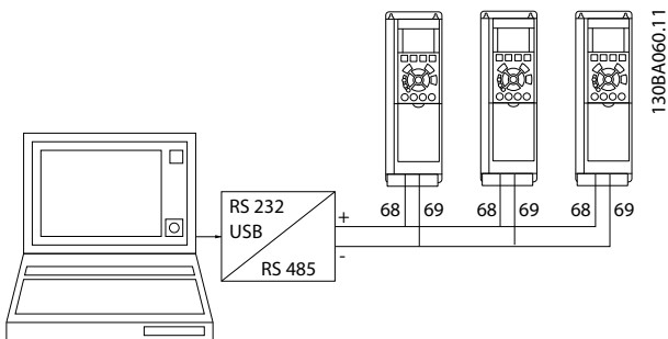
Abbildung 12.2 Parallele Verdrahtung
