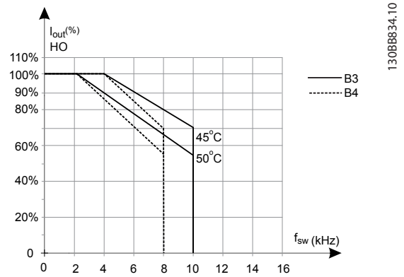
Abbildung 6.12 Leistungsreduzierung von I_{out} für abweichende T_{AMB, MAX} für die Bauformen B3 und B4, mittels SFAVM im Modus „Hohe Überlast“ (160 % Übermoment)
