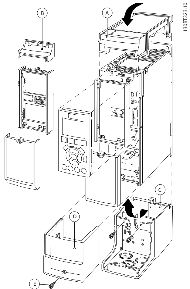
Abbildung 11.23 Baugröße A2
