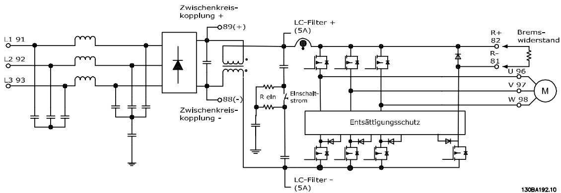
Abbildung 3.4 Steuerverfahren FC 301
