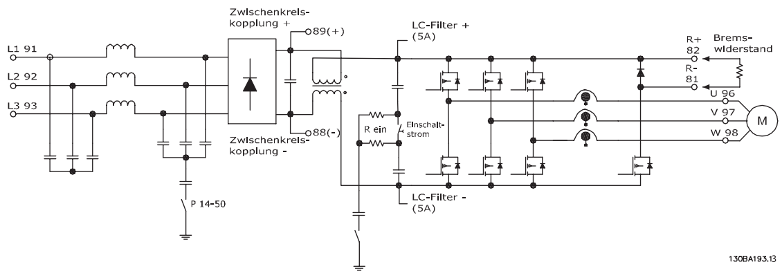
Abbildung 3.5 Steuerverfahren FC 302
