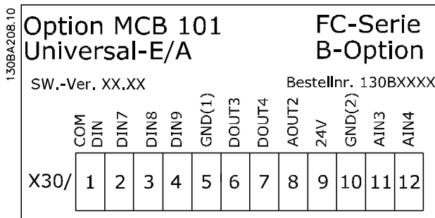
Abbildung 11.1 MCB 101-Option
