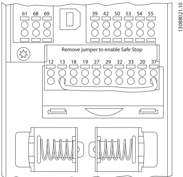
Abbildung 12.3 Steuerkartenklemmen
