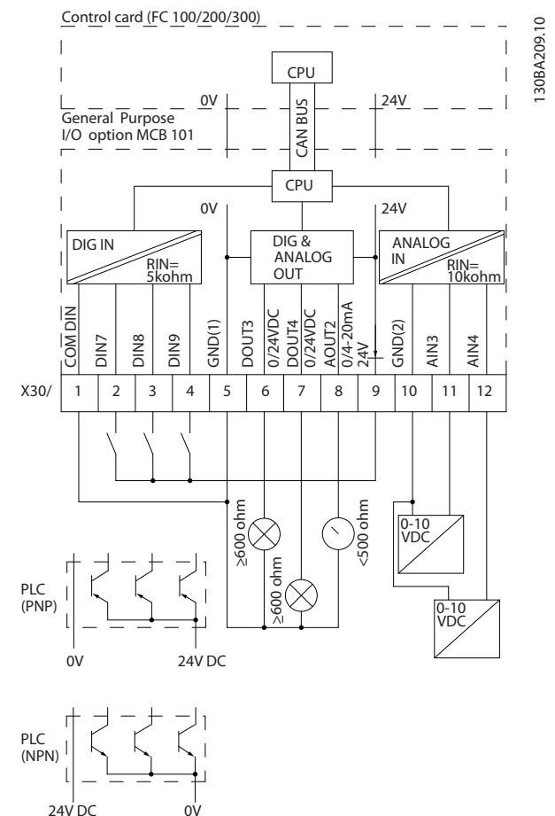
Abbildung 11.2 Prinzipschema
