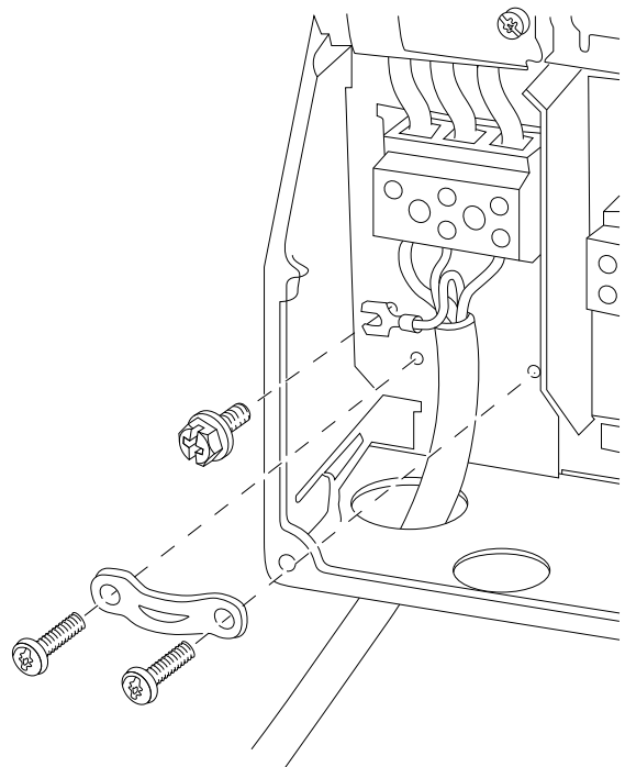
Abbildung 9.23 Netzanschluss Baugrößen B1 und B2
