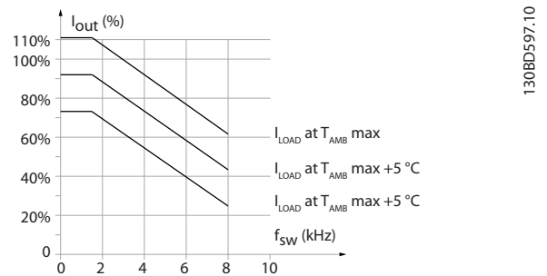
Abbildung 6.34 Leistungsreduzierung des Ausgangsstroms mit einer Schaltfrequenz und Umgebungstemperatur für Baugröße C3
