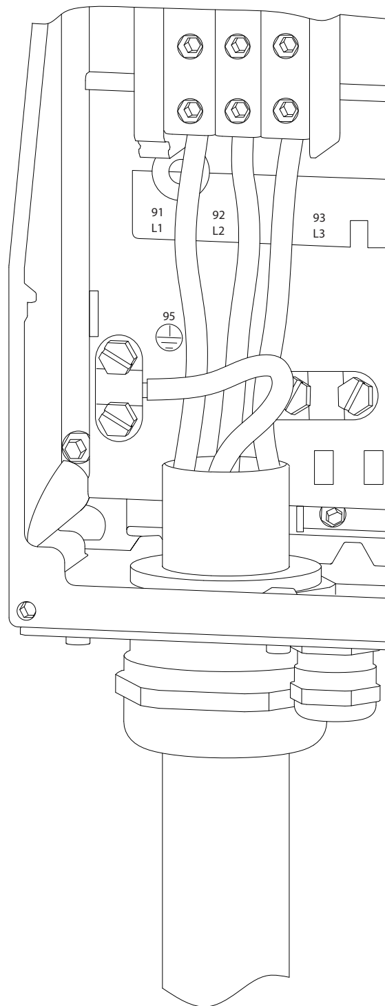
Abbildung 9.26 Netzanschluss Baugrößen C1 und C2 (IP21 und IP55/66).
