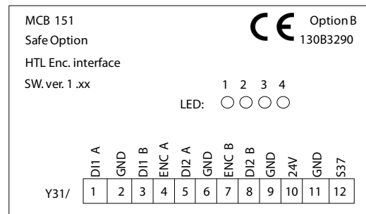
Abbildung 11.21 MCB 151
