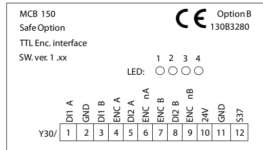
Abbildung 11.20 MCB 150
