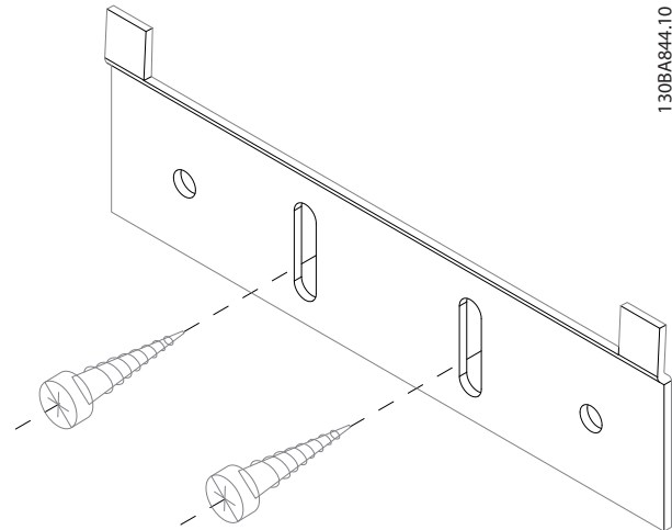
Abbildung 11.30 Untere Halterung
