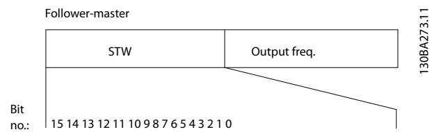
Abbildung 12.17 Zustandswort
