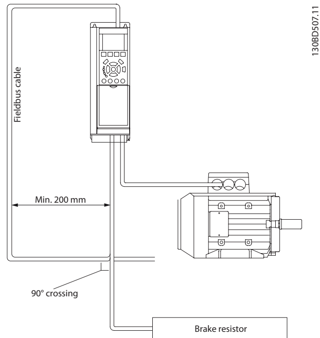
Abbildung 12.4 Kabelführung
