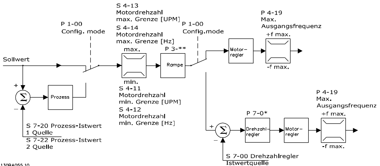
Abbildung 3.6 Regelungsstruktur bei VVC+-Konfigurationen mit und ohne Rückführung
