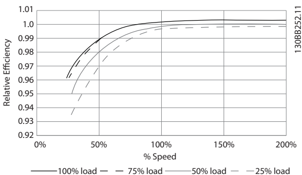
Abbildung 6.35 Typische Wirkungsgradkurven
