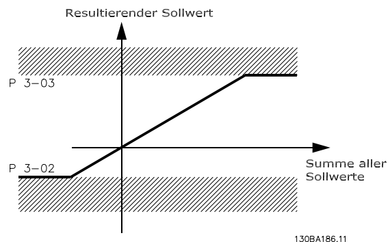
Abbildung 3.16 Summe aller Sollwerte bei Einstellung von 1-00 Regelverfahren auf [3] PID-Regler
