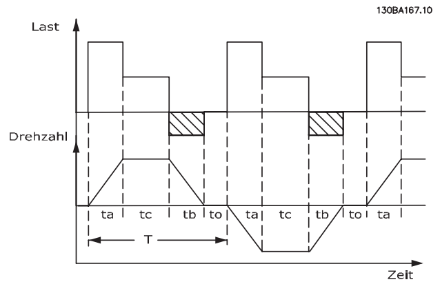
Abbildung 5.8 Typischer Bremszyklus
