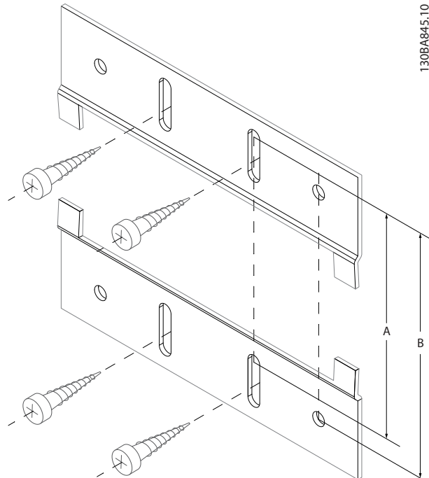
Abbildung 11.31 Obere Halterung
