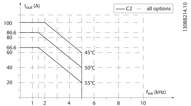
Abbildung 6.33 Leistungsreduzierung des Ausgangsstroms mit einer Schaltfrequenz und Umgebungstemperatur für Baugröße C2, SFAVM. Bemerkung: Die Kurve wird mit dem Strom als Absolutwert gezeichnet und gilt sowohl für hohe als auch normale Überlast.
