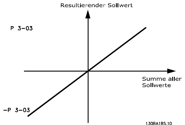
Abbildung 3.15 Resultierender Sollwert
