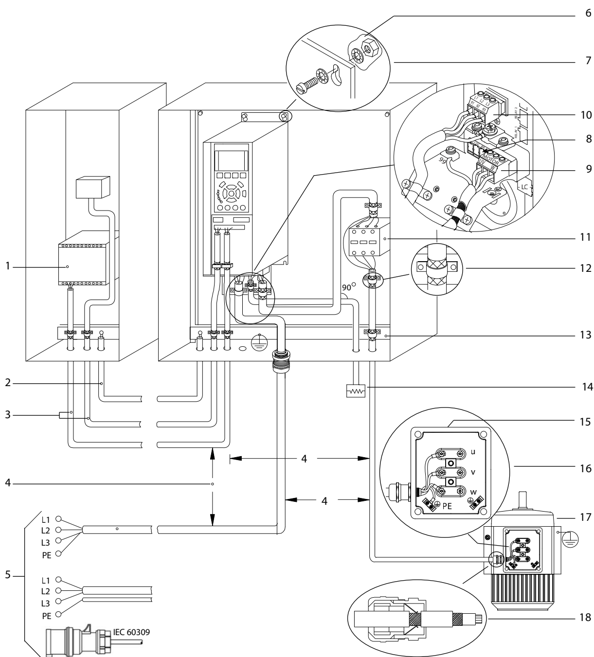
Abbildung 28: Typische elektrische Verbindung
