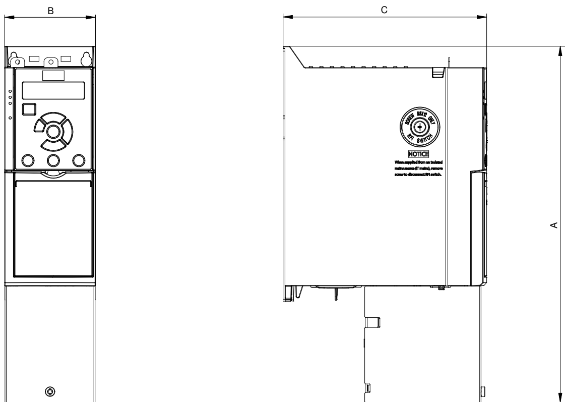
Abbildung 17: Standard mit unterer Kabeleinführungsabdeckung (ohne obere Abdeckung)
