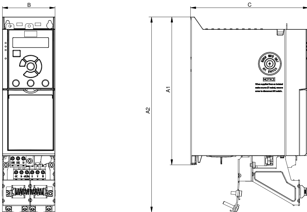
Abbildung 16: Standard mit Abschirmblech
