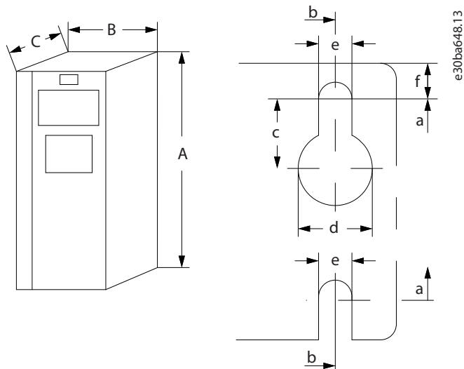
Abbildung 19: Befestigungsbohrungen oben und unten
