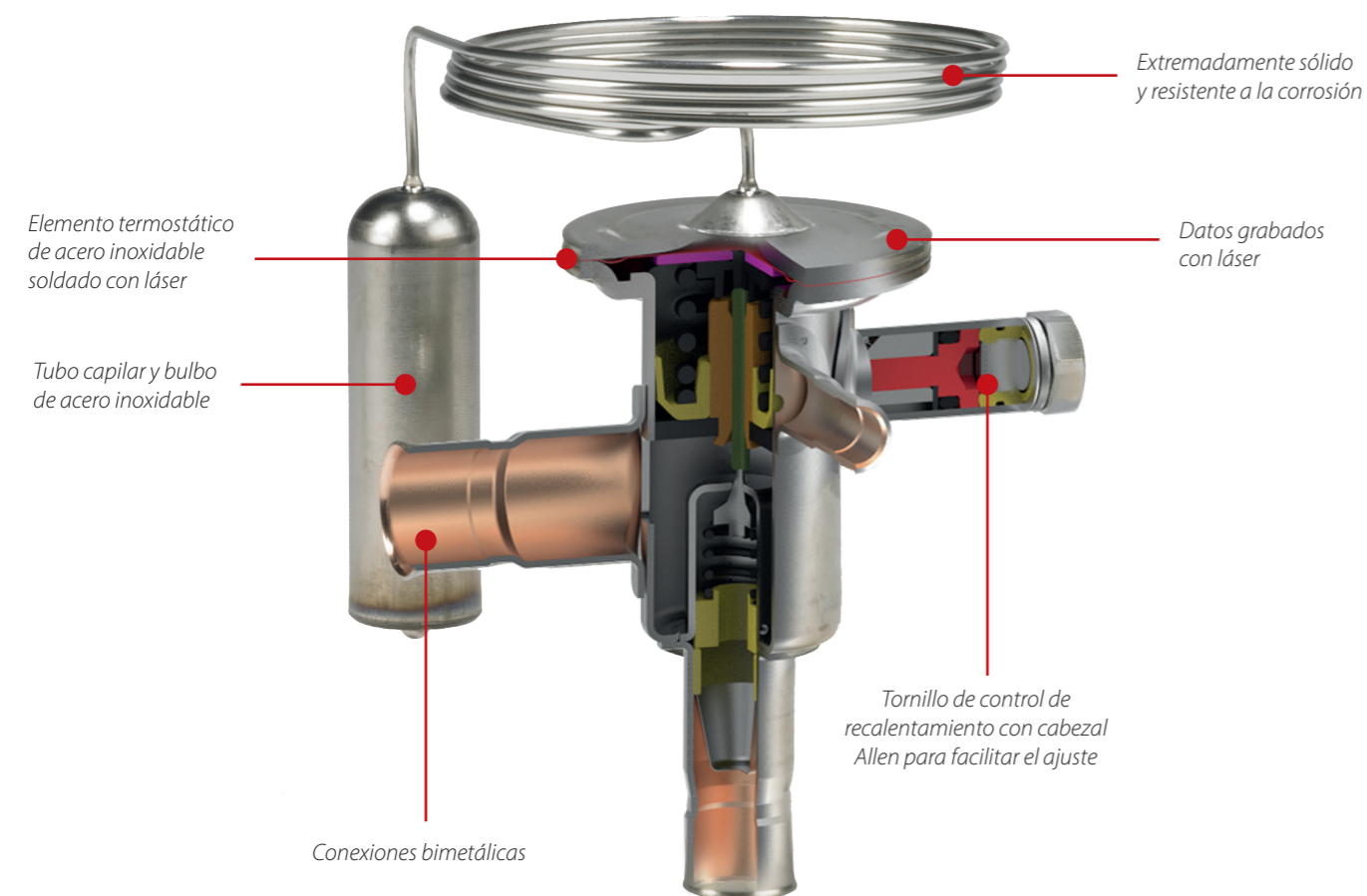
Válvula de expansión termostática TUBE
