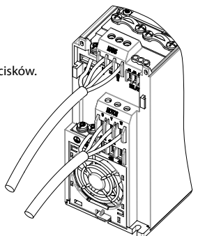
Ilustracja 1: Montaż kabla uziemienia, zasilania i przewodów silnika
