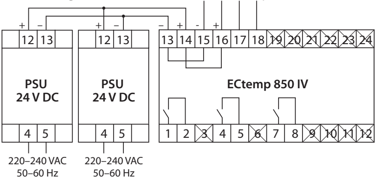
**Fig. H — connexion de 2 modules en parallèle
