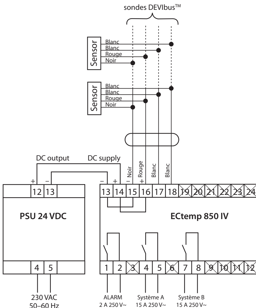
Fig. A — Connexion du ECtemp 850 IV
