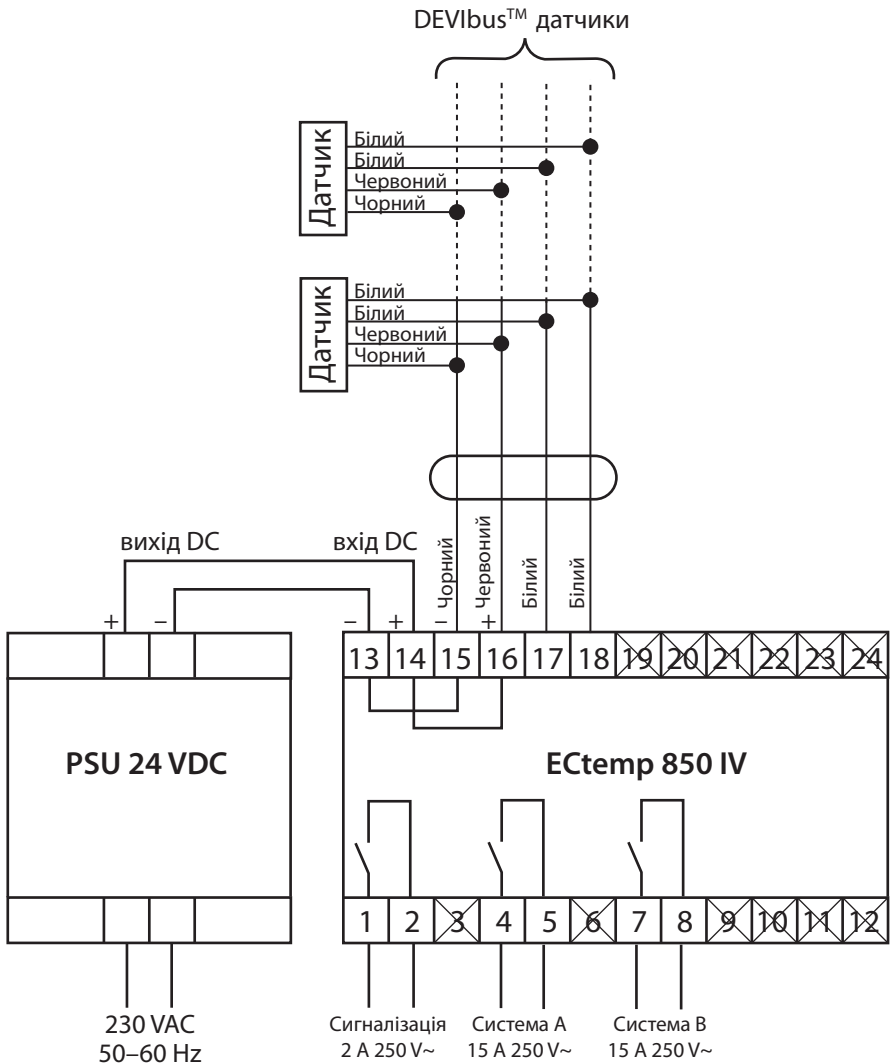
Рис. А — Підключення ECtemp 850
