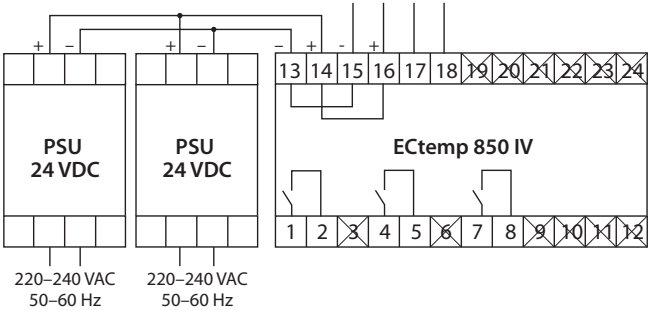
**Рис. Н — з'єднання 2 блоків живлення (PSU) в паралель
