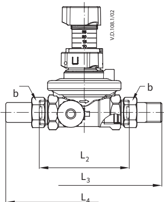
外螺纹 (ISO 228/1)
