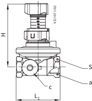
内螺纹 (ISO 7/1)
