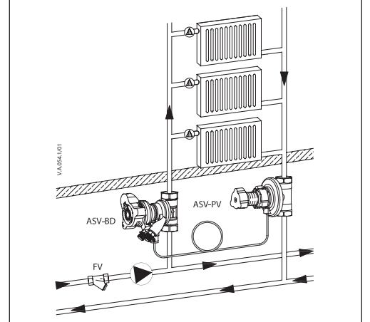
Şek. 3 ASV dikey kolon / tipik radyatör ısıtma uygulamasında (genel örnek)
