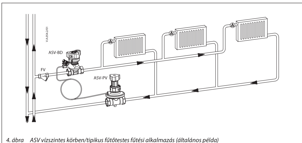
4. ábra ASV vízszintes körben/tipikus fűtőtestes fűtési alkalmazás (általános példa)
