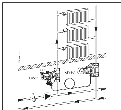
3. ábra ASV a függőleges ágba/tipikus fűtőtestes fűtési alkalmazás (általános példa)
