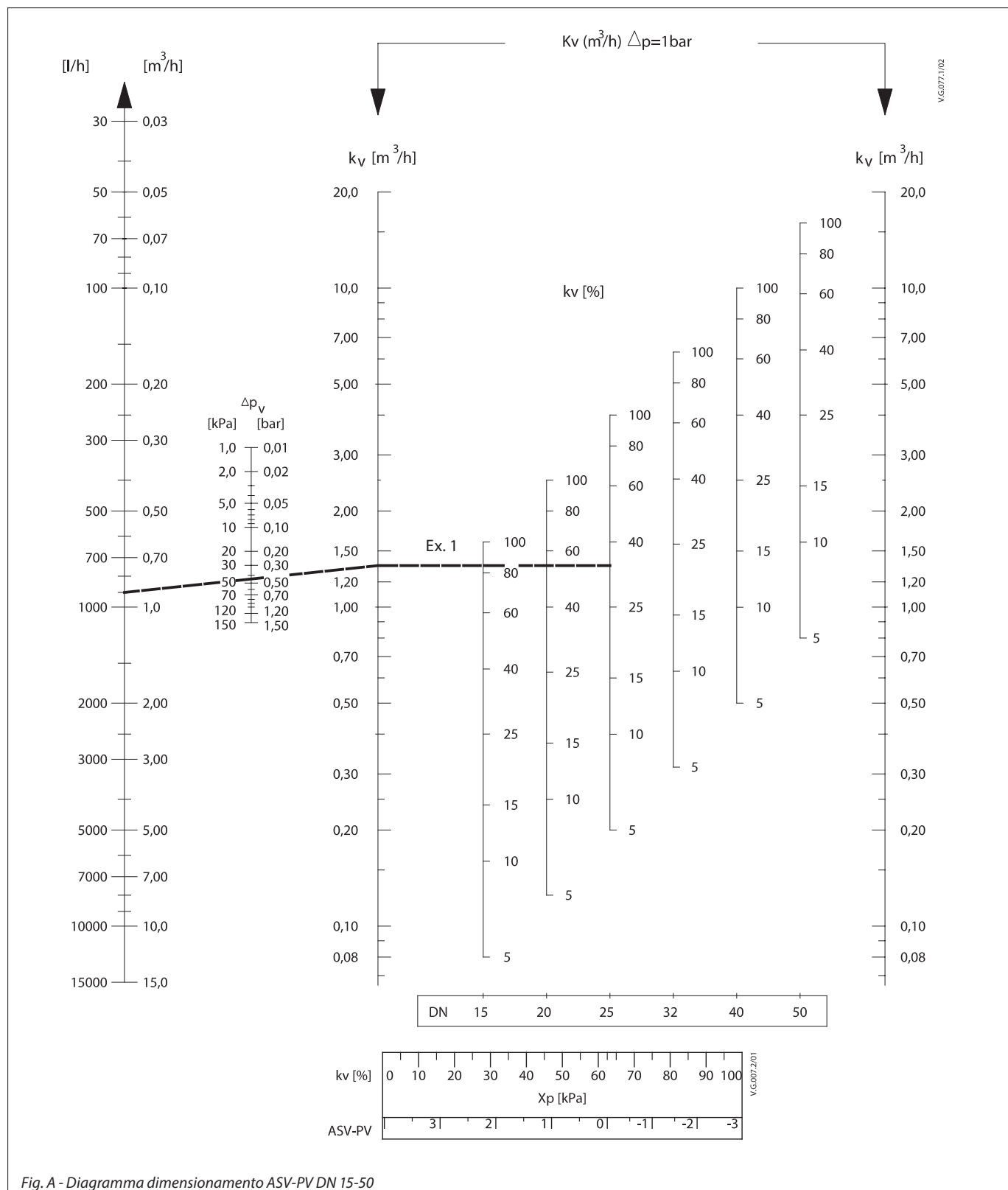
Fig. A - Diagramma dimensionamento ASV-PV DN 15-50
