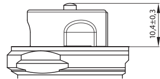
Punto di chiusura (misurazione) per DN 15-32
