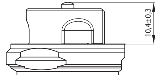
Punkt zamknięcia (pomiar) dla DN 15-32
