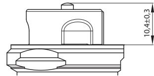
Point de fermeture (mesure) pour DN 15-32
