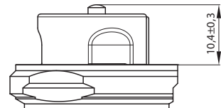
Zaporna točka (mera) za DN 15–32
