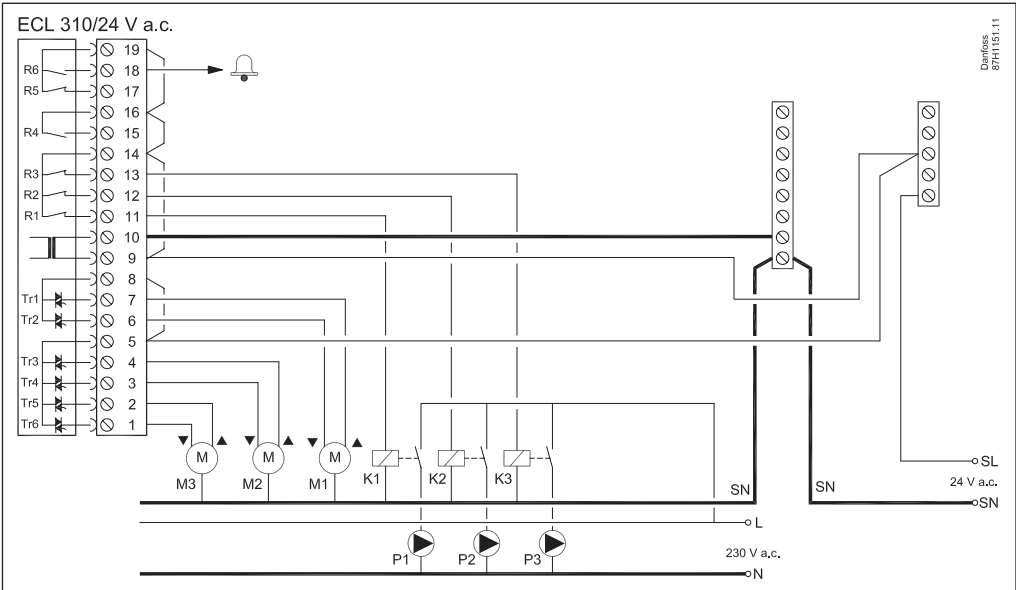
ECL Comfort 310 vadojuma piemērs
