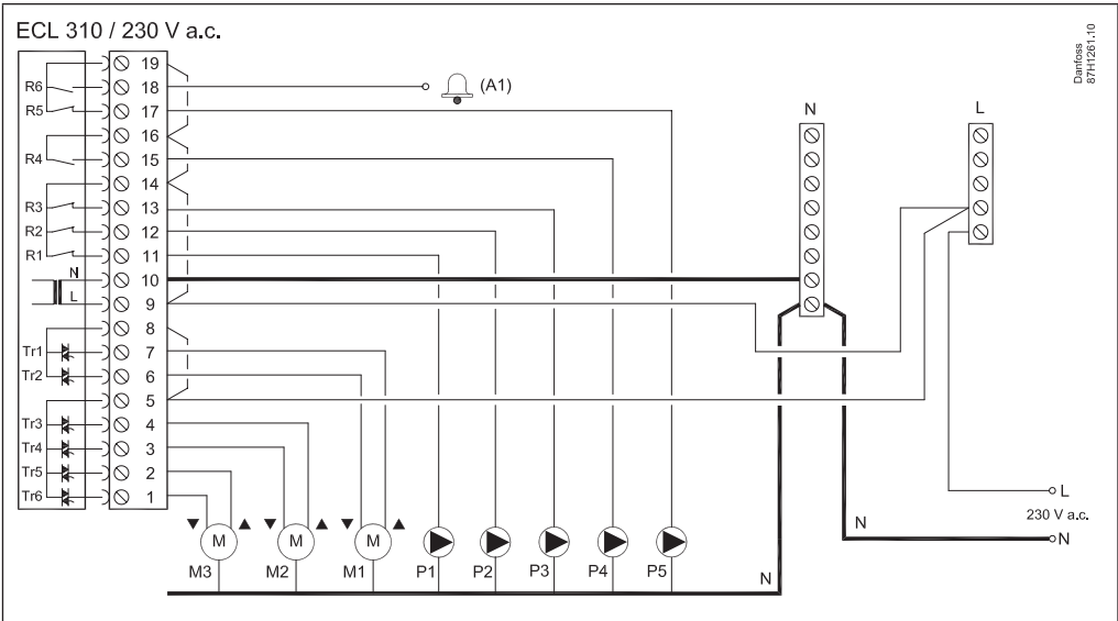
ECL Comfort 310 vadojuma piemērs
