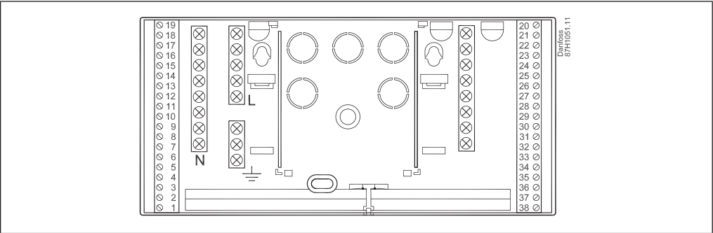
ECL Comfort 310 pamatdaļa (to var izmantot arī regulatoram ECL Comfort 210).
