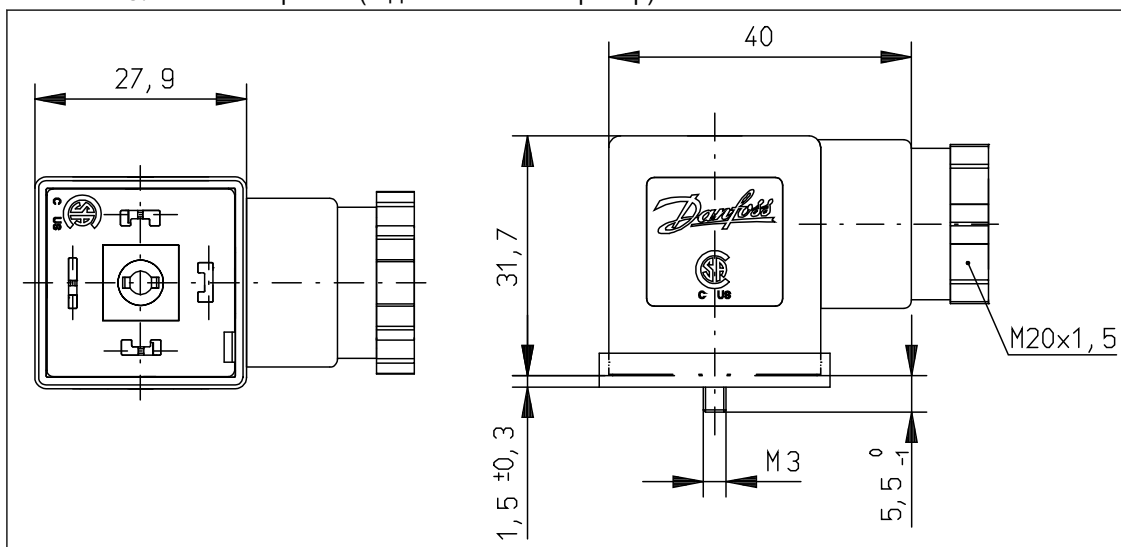
Малюнок 45: Кабельний роз'єм (Підсвітка LED + Варістор)
