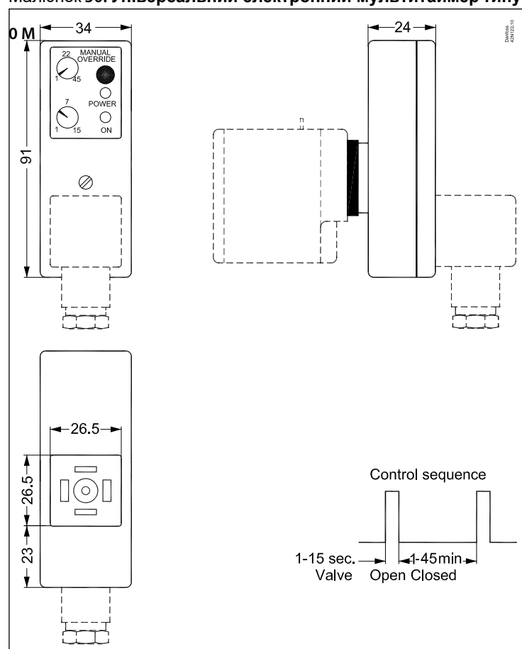
Малюнок 50: Універсальний електронний мультитаймер типу ET 2
