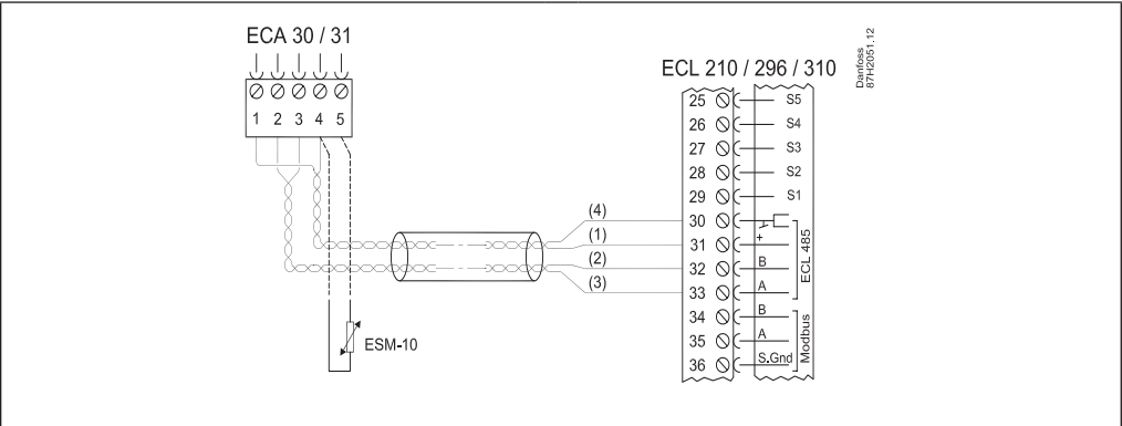
Verdrahtung des ECL Comfort 296 und der ECA 30/31
