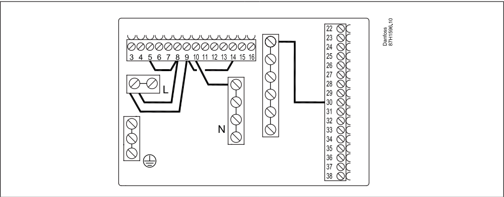
Sockel für den ECL Comfort 296 mit Vorverdrahtung
