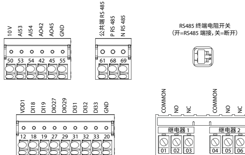
图 4: 控制端子
