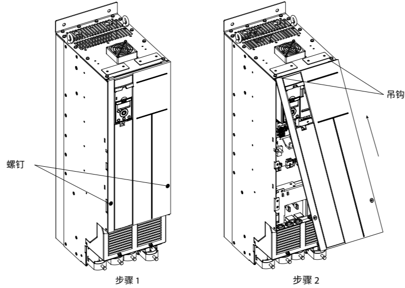
图 2: 拆除前盖
