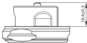
关闭点 (测量) 适用于 DN 15-32
