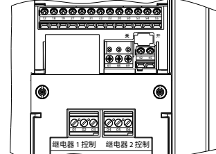
图 4: 控制端子及继电器连接 (机箱规格 J6–J7)
