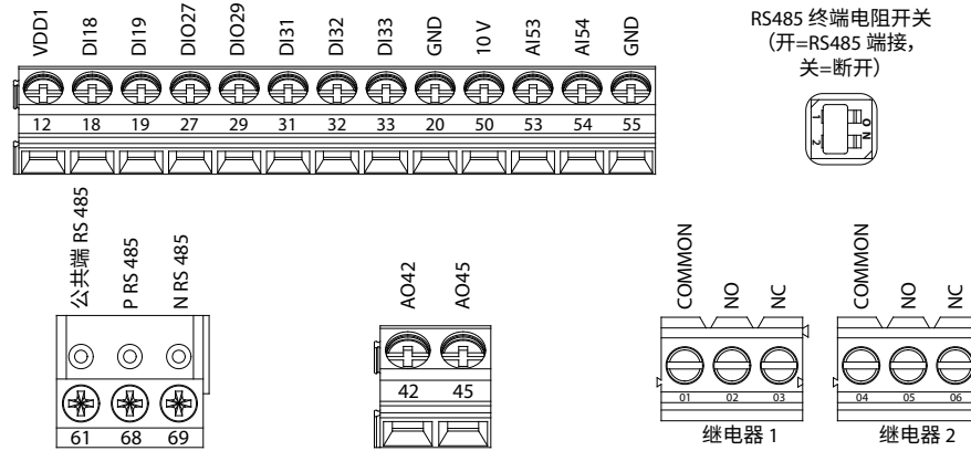
图 7: 控制端子
