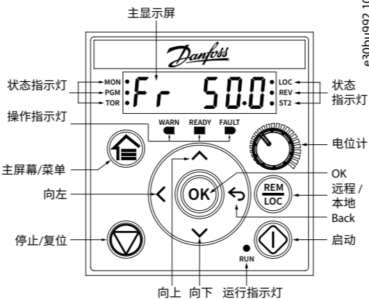
图 5: 指示灯和操作按钮
