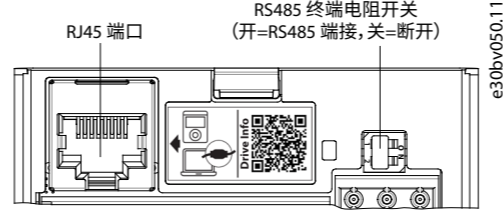
图 4: RJ45 端口和 RS485 端接开关
