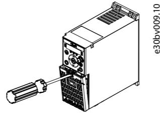
图 2: 拆除端子盖
