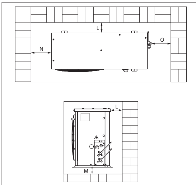
Abbildung 1: Mindestmontageabstände
