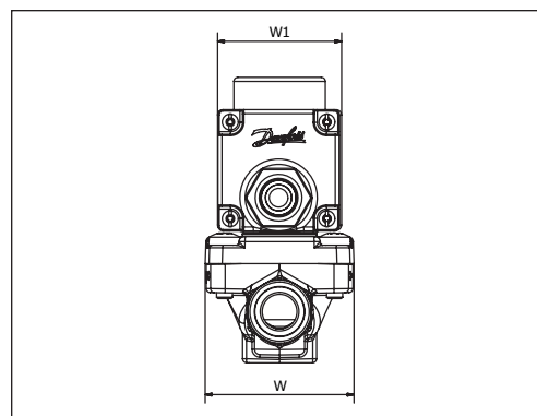
Вид сбоку
