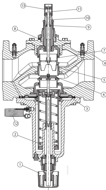
Abb. 14: AB-PM DN 65–100
