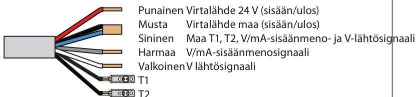
Sininen O-rengas
