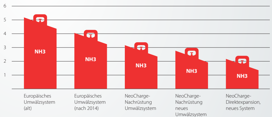
Ammoniakfüllmenge (kg/kW)
