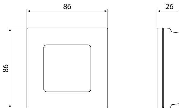
Bezdrátový prostorový termostat Danfoss Icon™
