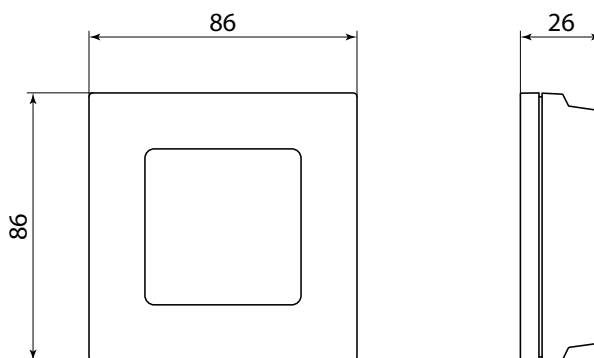
Bezdrôtový izbový termostat Danfoss Icon™
