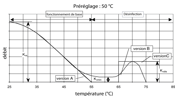
Fig.13 : caractéristiques de régulation de la MTCV
