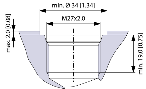
1C M27 x 2.0 ISO 6149-1
