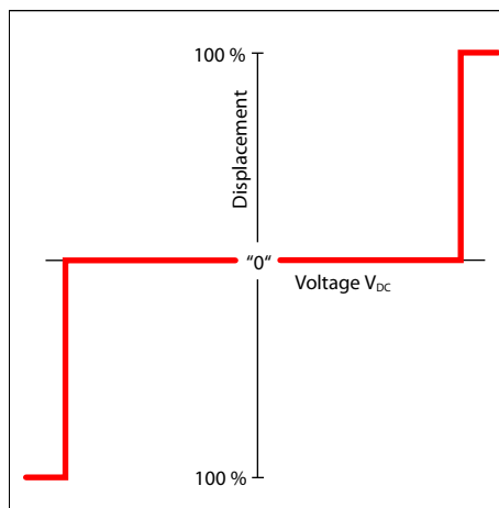
ポンプ容量と電気信号
