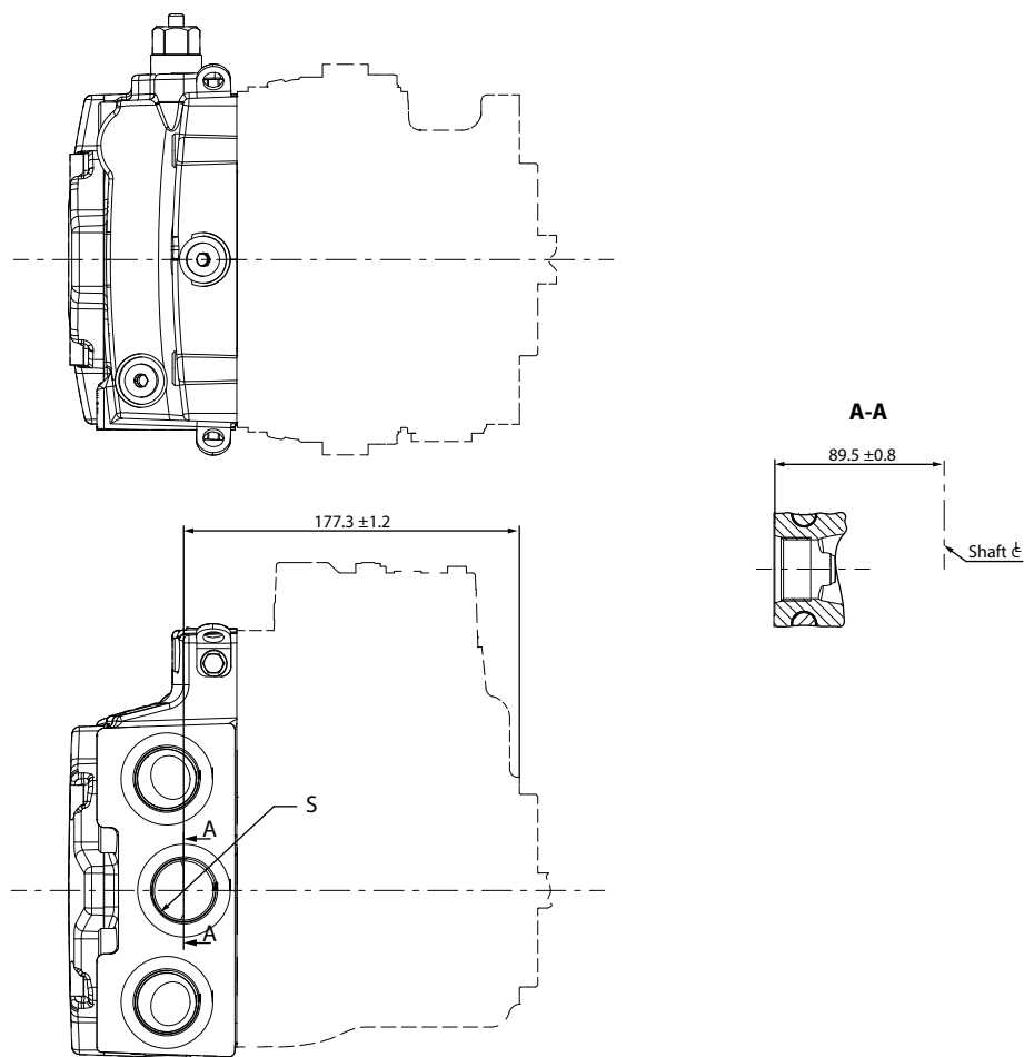
S ISO 1926-1 に基づくチャージ入口ポート; 1 5/16-12
