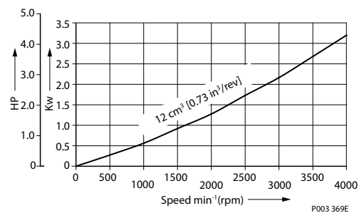
必要チャージポンプ動力
