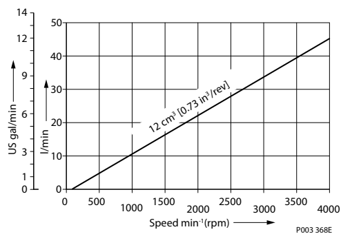
チャージポンプ流量
