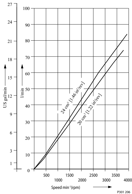
チャージポンプ流量
