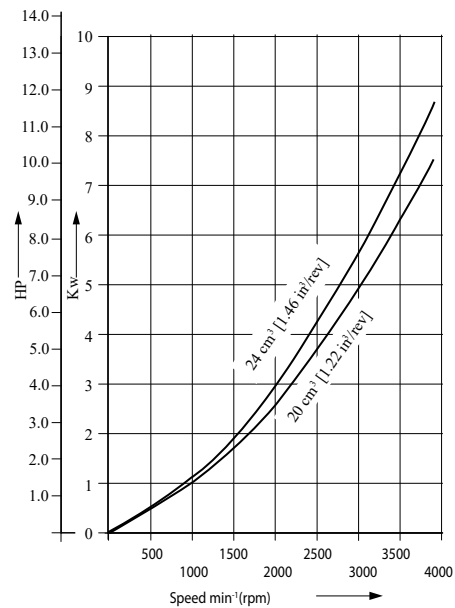
必要チャージポンプ動力
