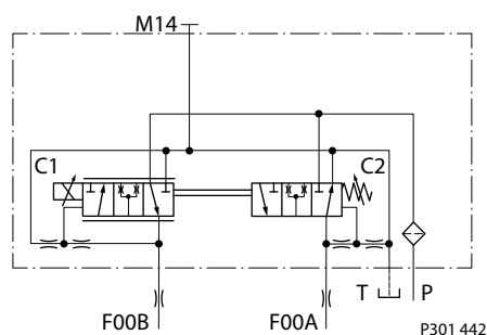
FDC 回路図
