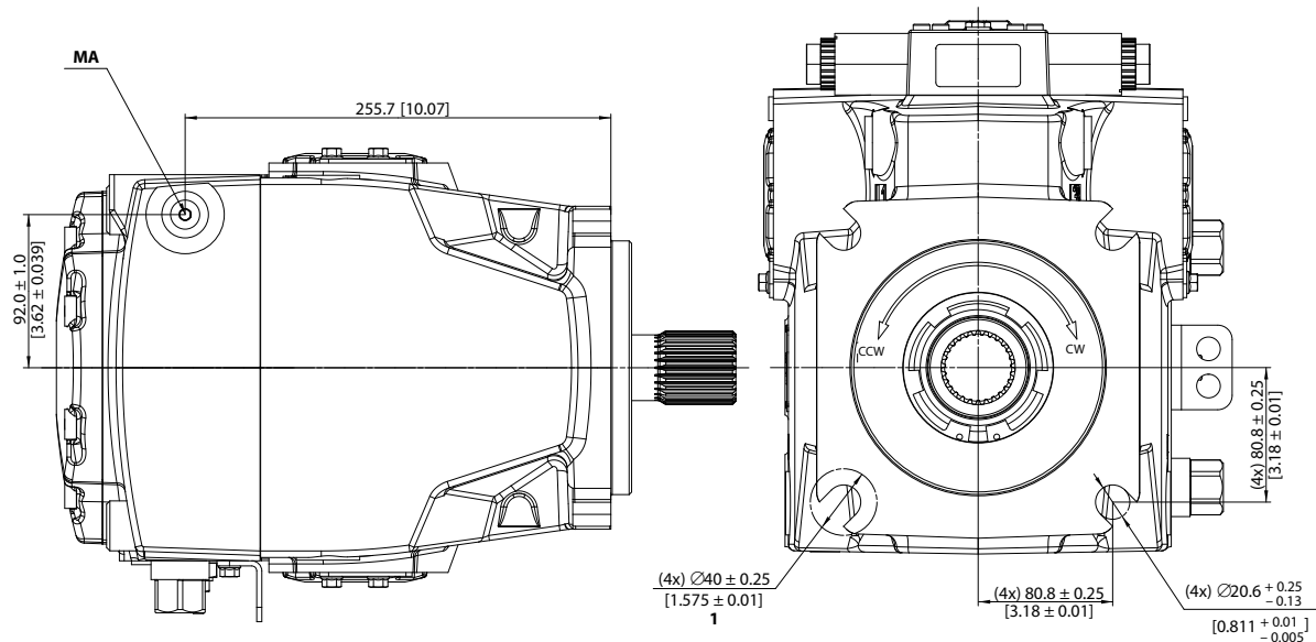
1 — 反対側のねじ頭スペース
