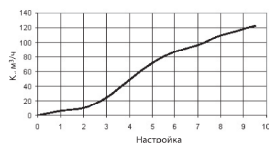
Расходная характеристика
