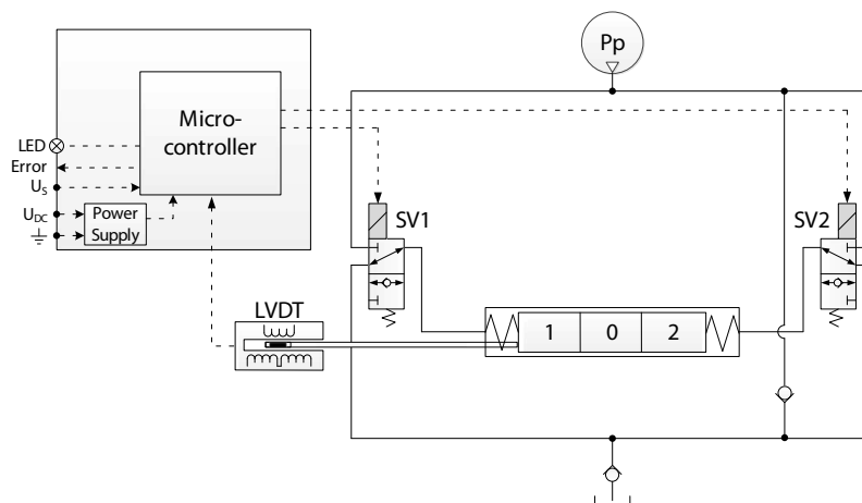
高速応答性機能付 PVEM (PVEM-Q) 機能ダイアグラム
