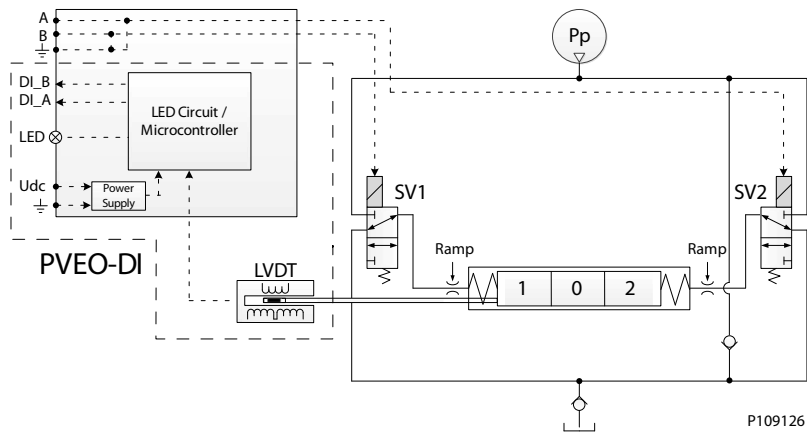
PVEA-DI 機能ダイアグラム
