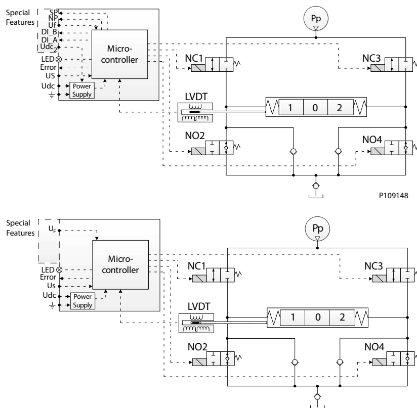
PVEH-FLA 機能ダイアグラム
