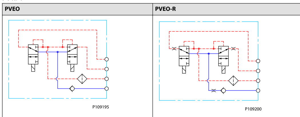
回路図
