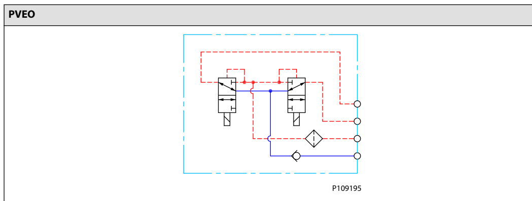
PVEO 回路図
